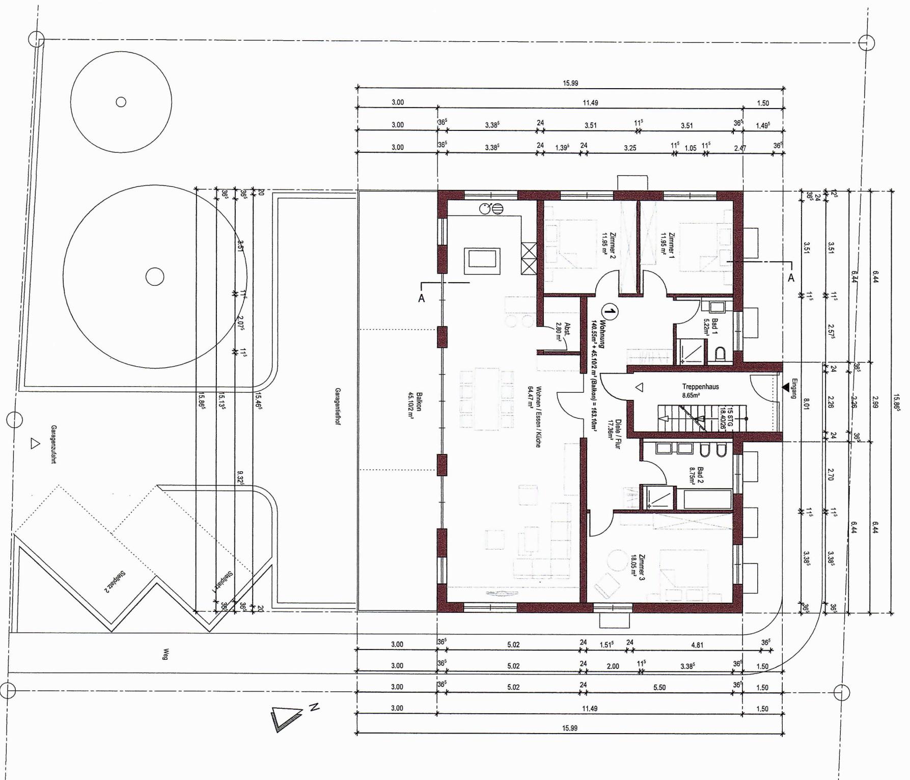
Grundriss Erdgeschoss
