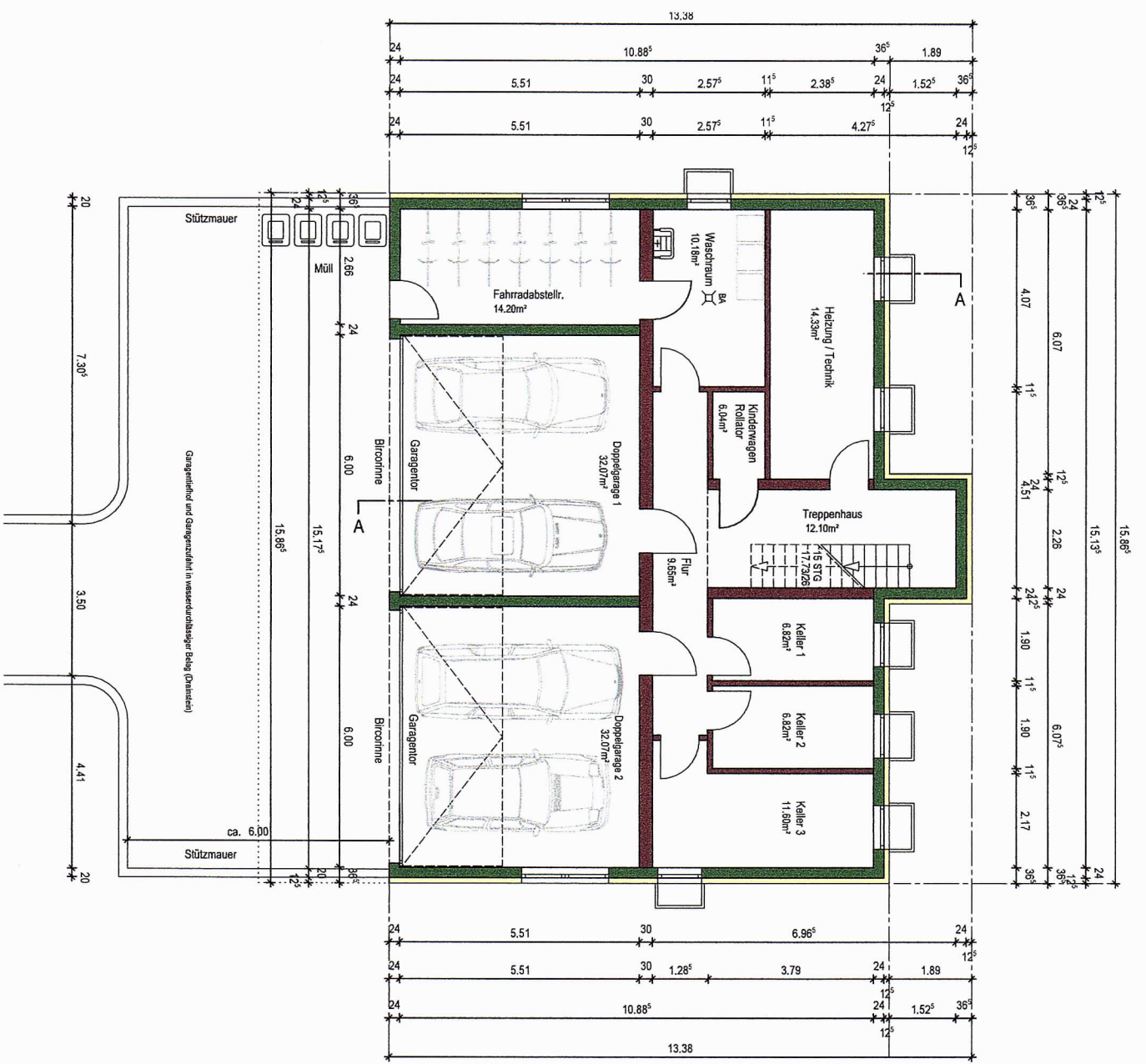
Grundriss Untergeschoss
