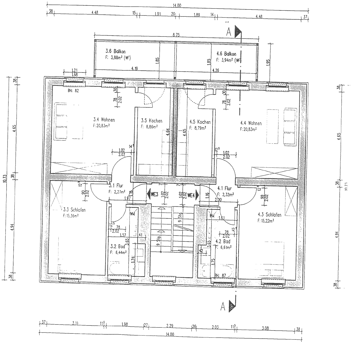
Grundriss 1.Obergeschoss
