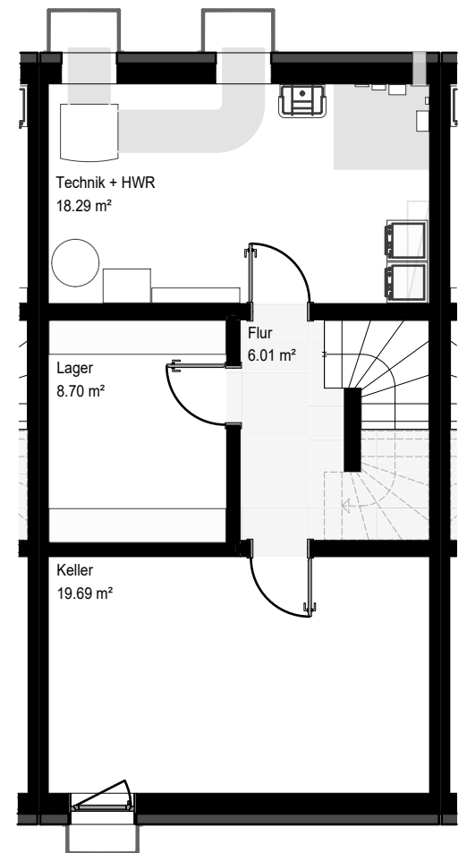
KELLERGESCHOSS
