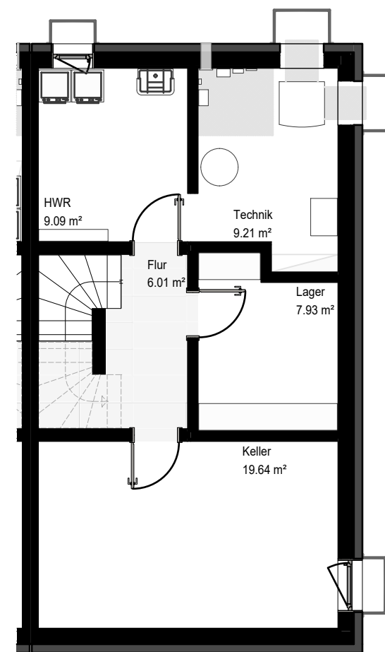
KELLERGESCHOSS
