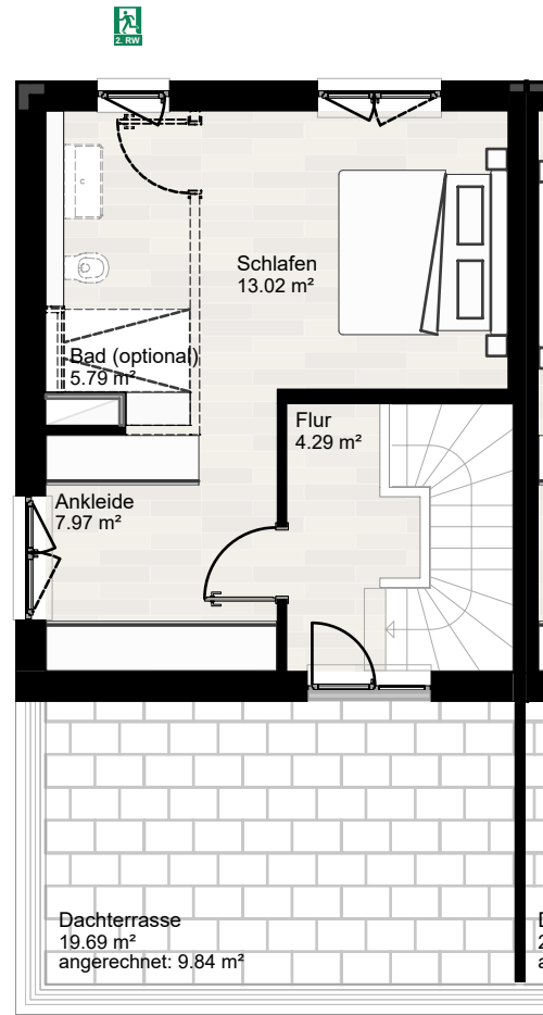
DACHGESCHOSS
