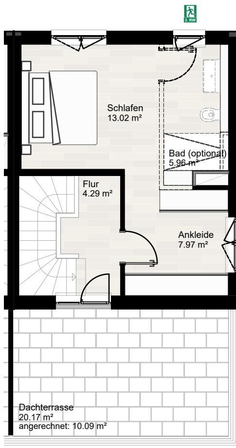
DACHGESCHOSS
