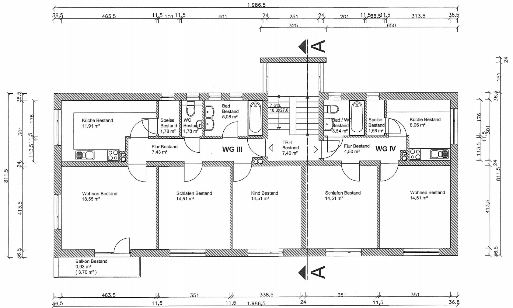
Grundriss 2. OG Bestand
