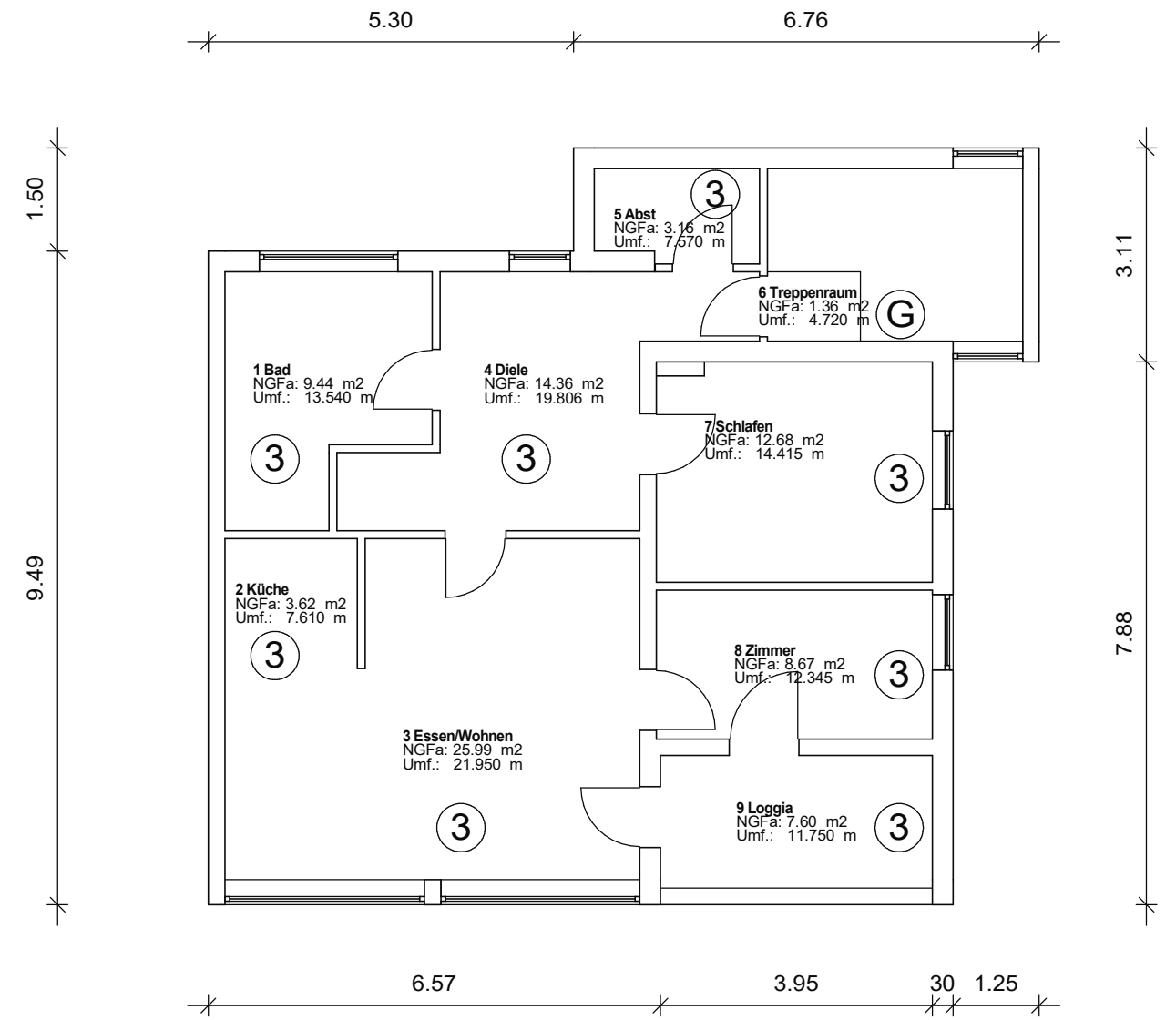
2. OBERGESCHOSS
