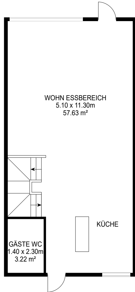
ERDGESCHOSS
