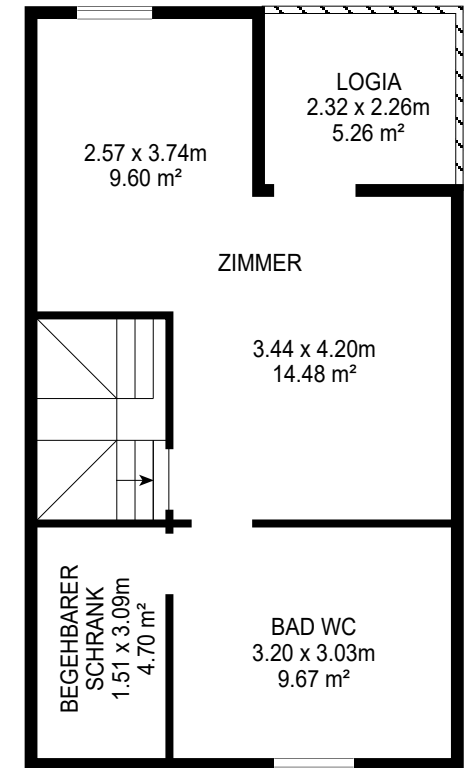
DACHGESCHOSS
