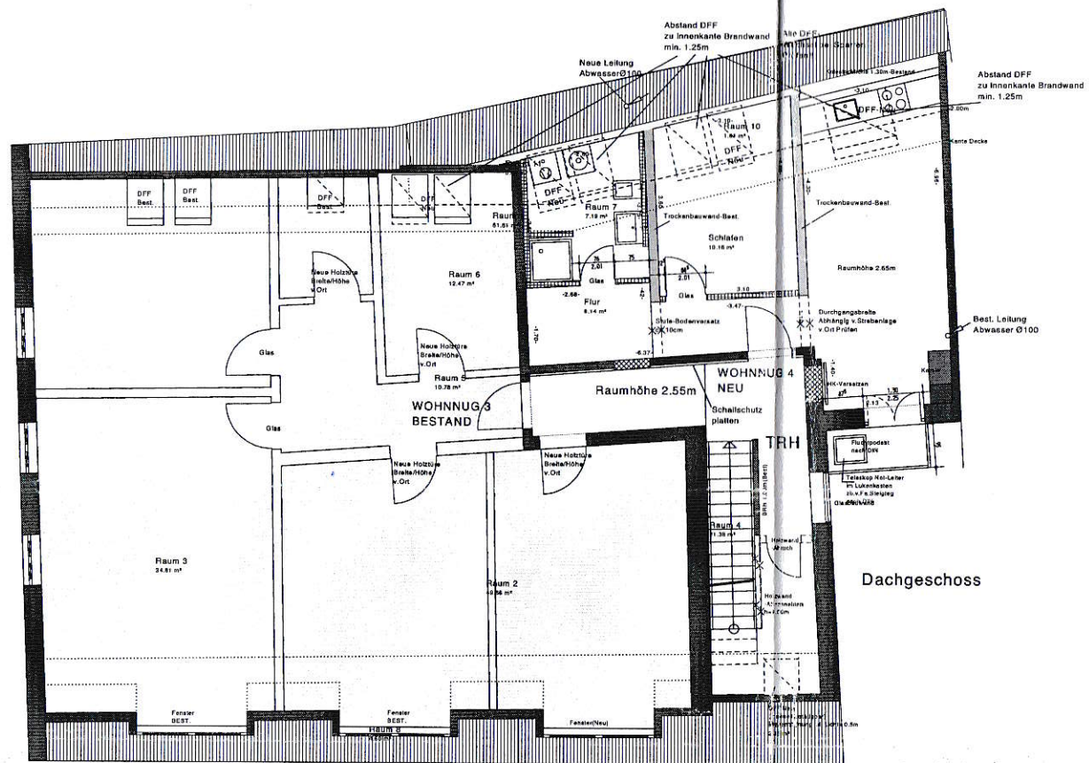
GRUNDRISS DACHGESCHOSS UMBAU
