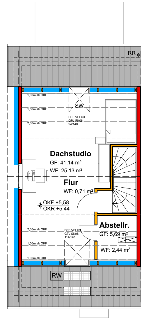
DACHGESCHOSS
