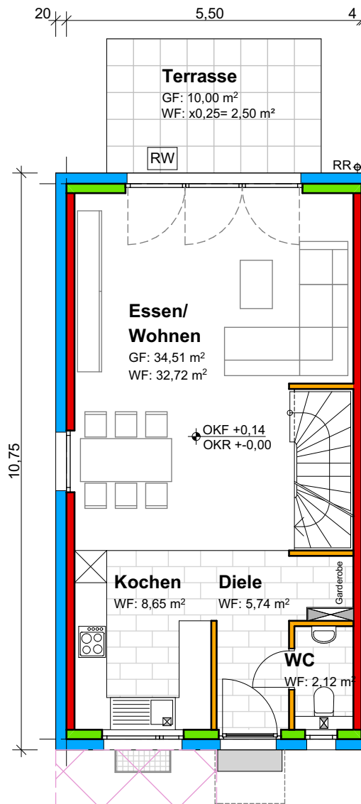
ERDGESCHOSS
