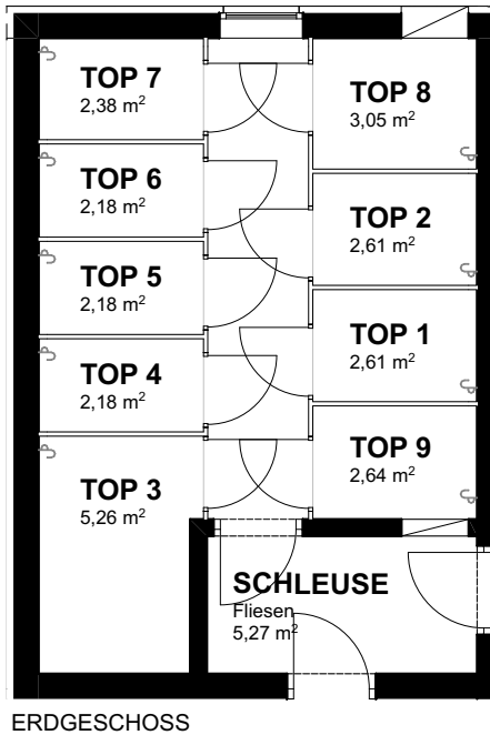
ERDGESCHOSS
