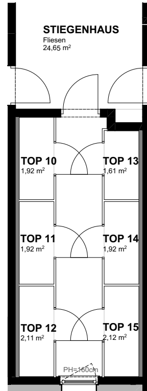
1.OBERGESCHOSS
