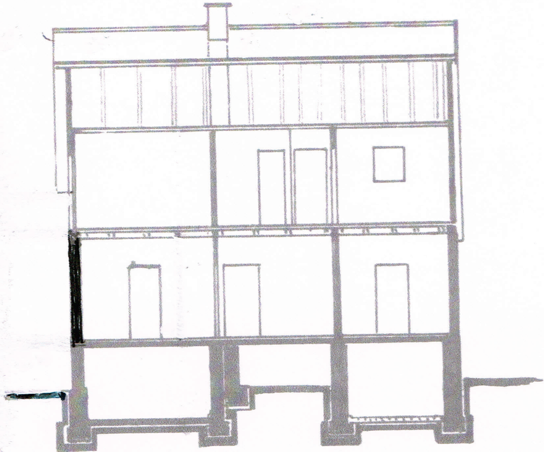
Schnitt: A-B.
