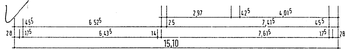
GRUNDRISS EG.
