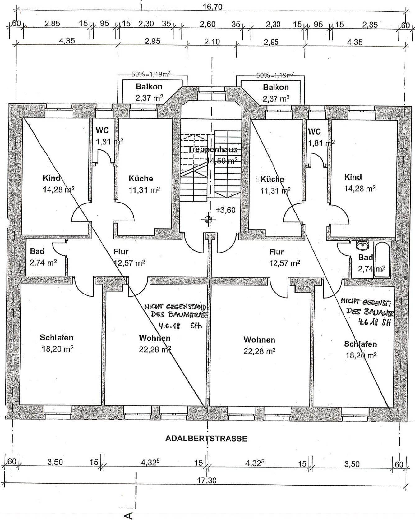
riss 1. OG - 3. OG Gegenstand der Baueingabe -
