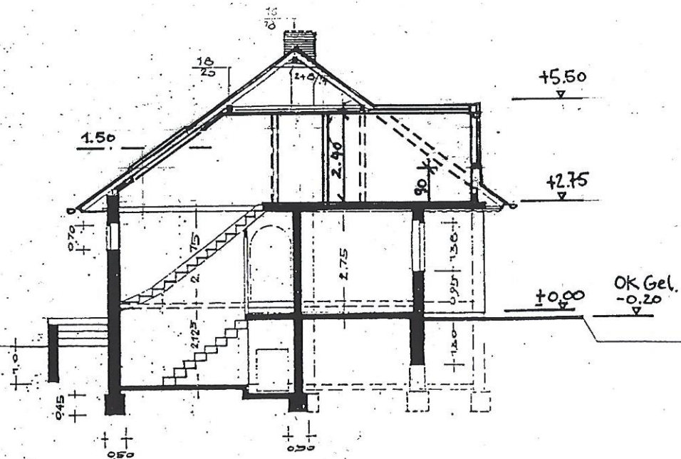
Schnitt 1 - 1 M 1:100
