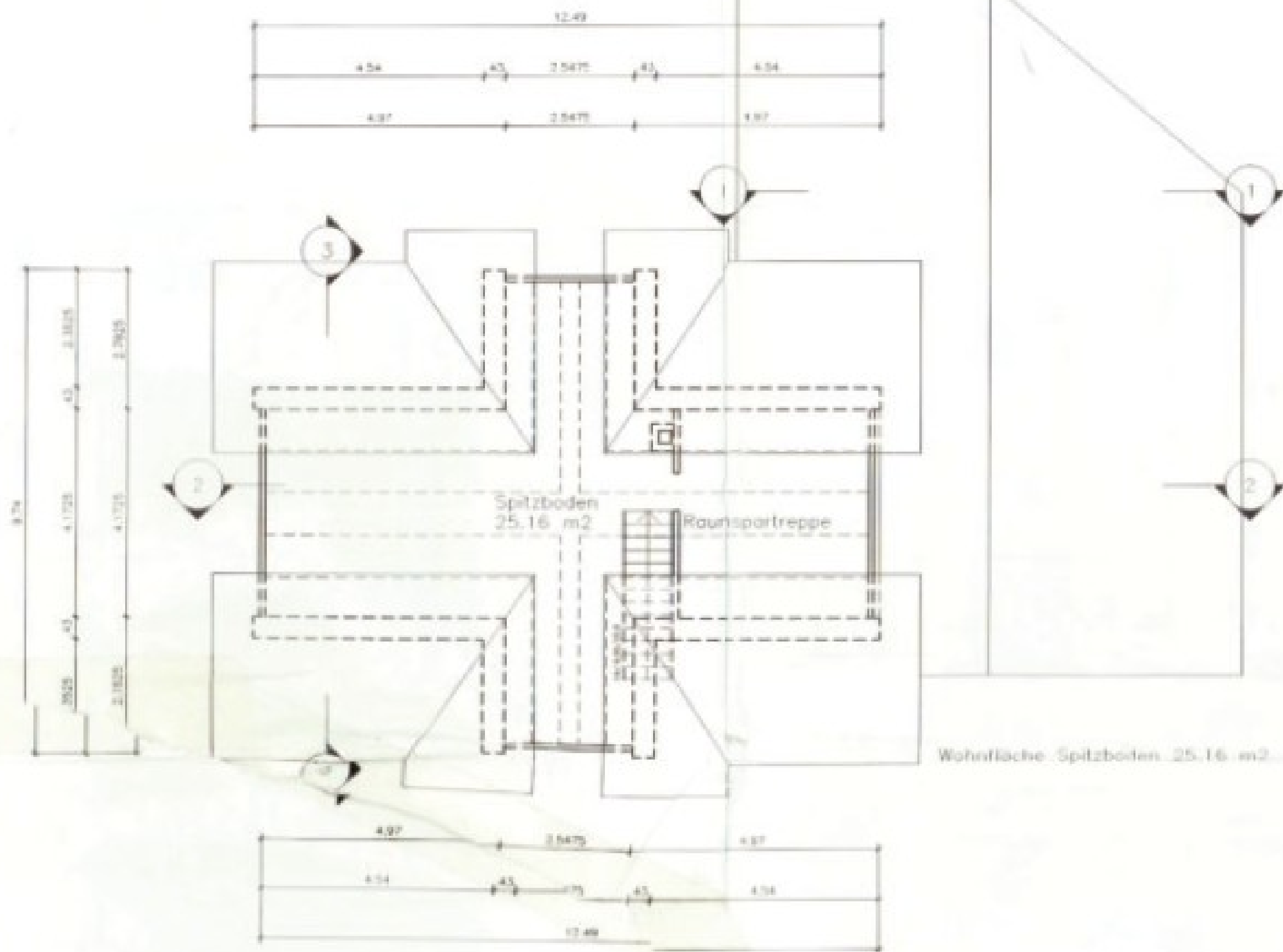
Grundriss Spitzboden
