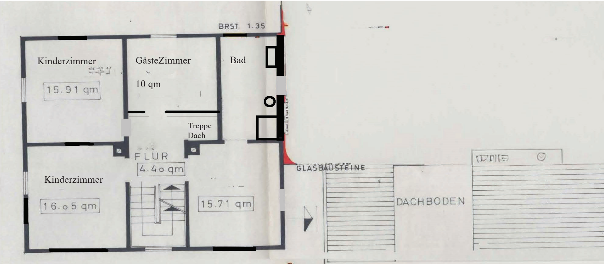
Grundrisse – Dachgeschoss - Haupthaus
