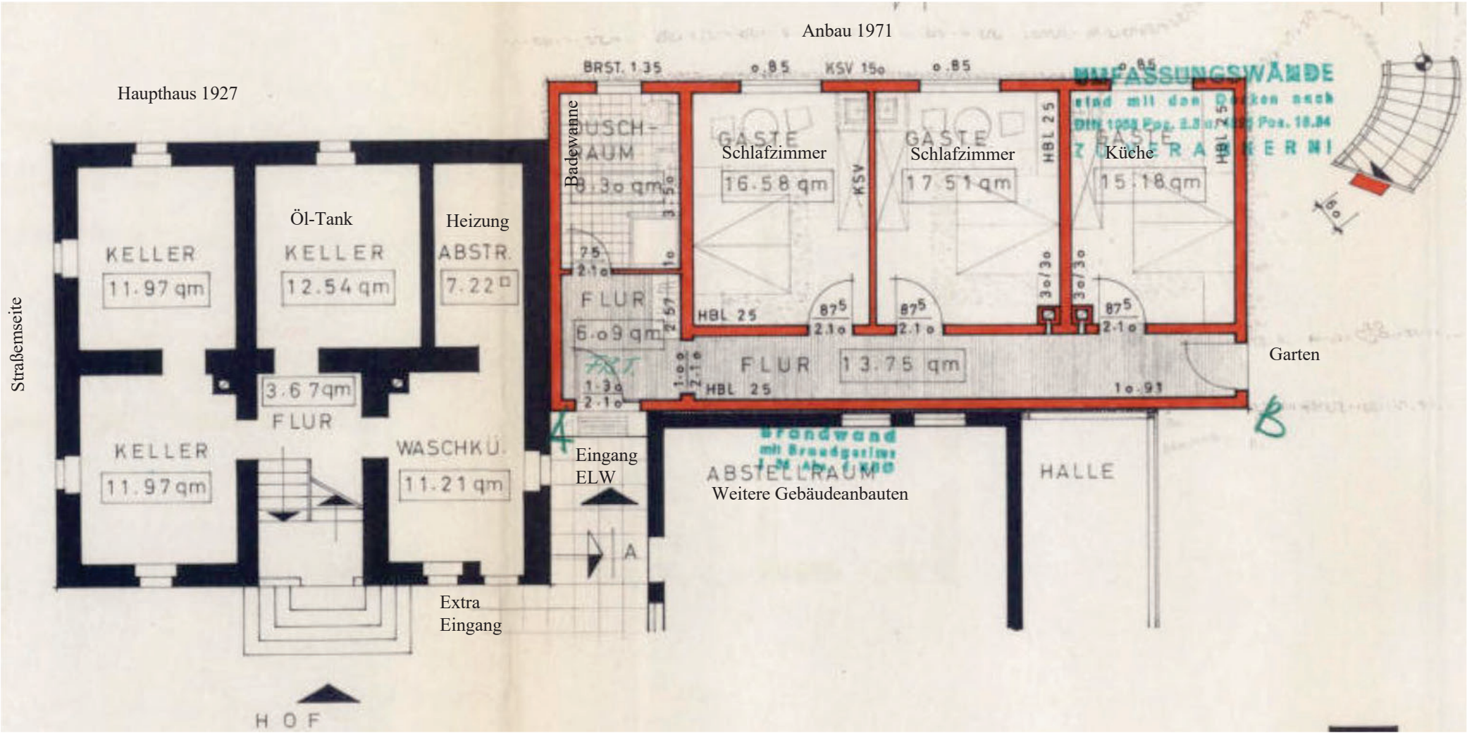
Grundrisse, Kellergeschoss Boden-Ebene wie Erdgeschoss
