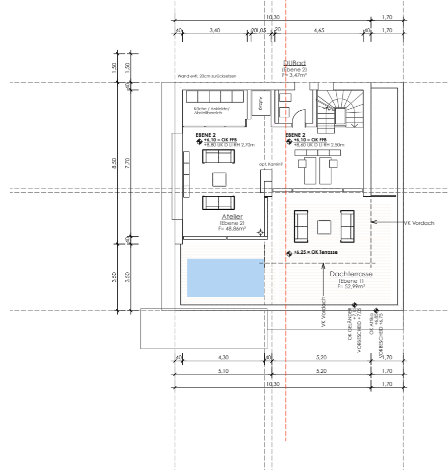
Haus B Grundriss EBENE 2
