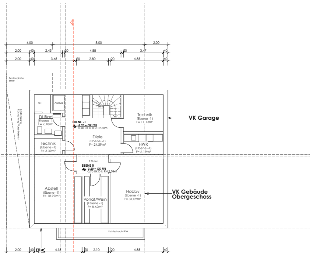
Haus B Grundriss EBENE -1
