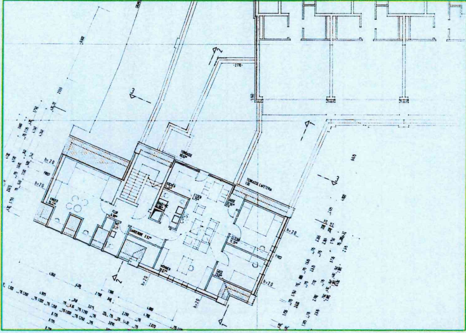
Übersichtsplan Dachgeschoß
