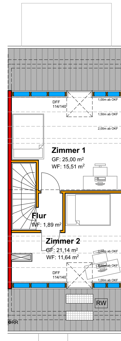
Dachgeschoss
