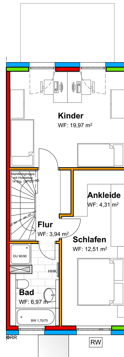
Obergeschoss
