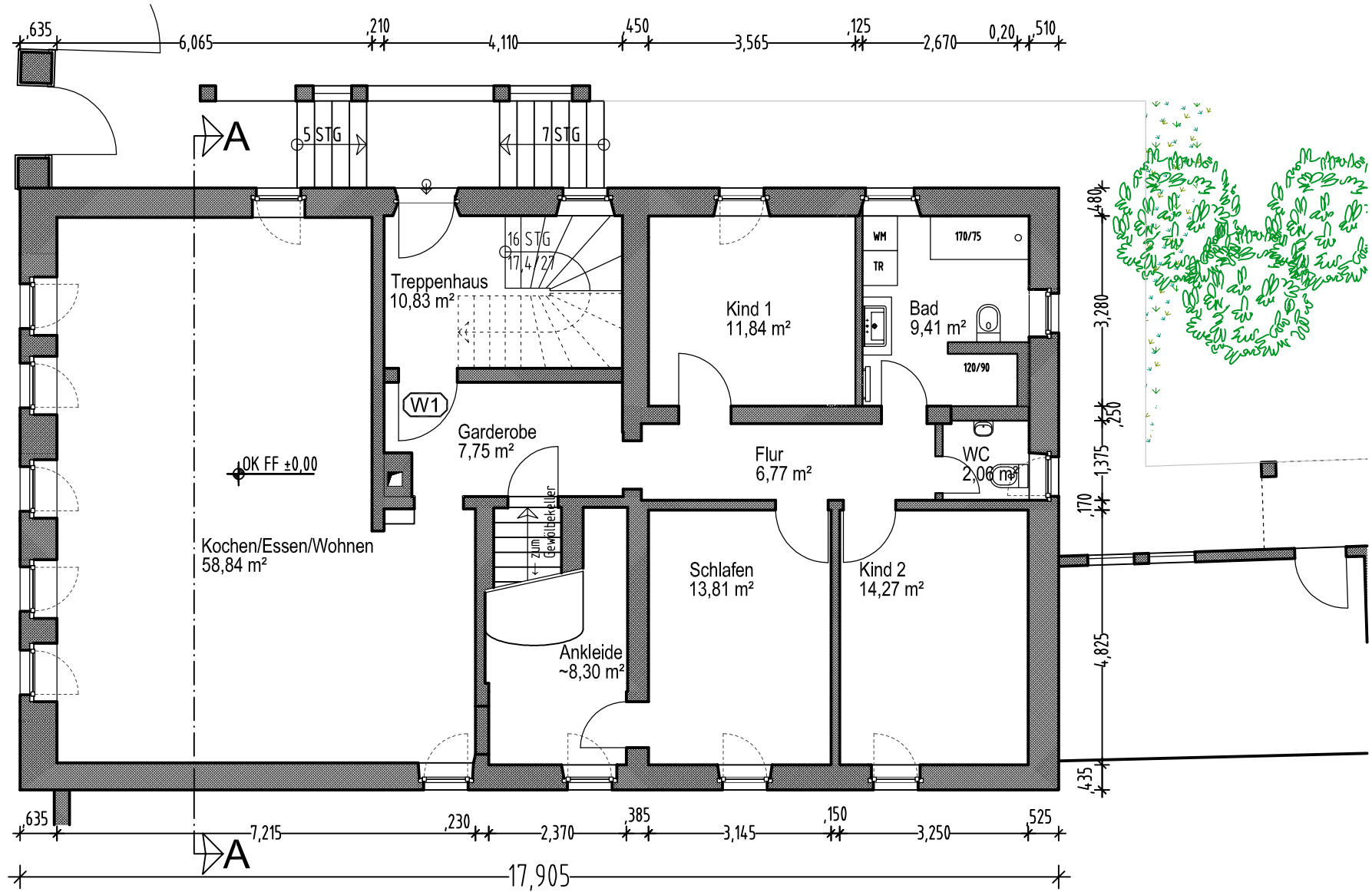
Grundriss EG M. 1 : 100
