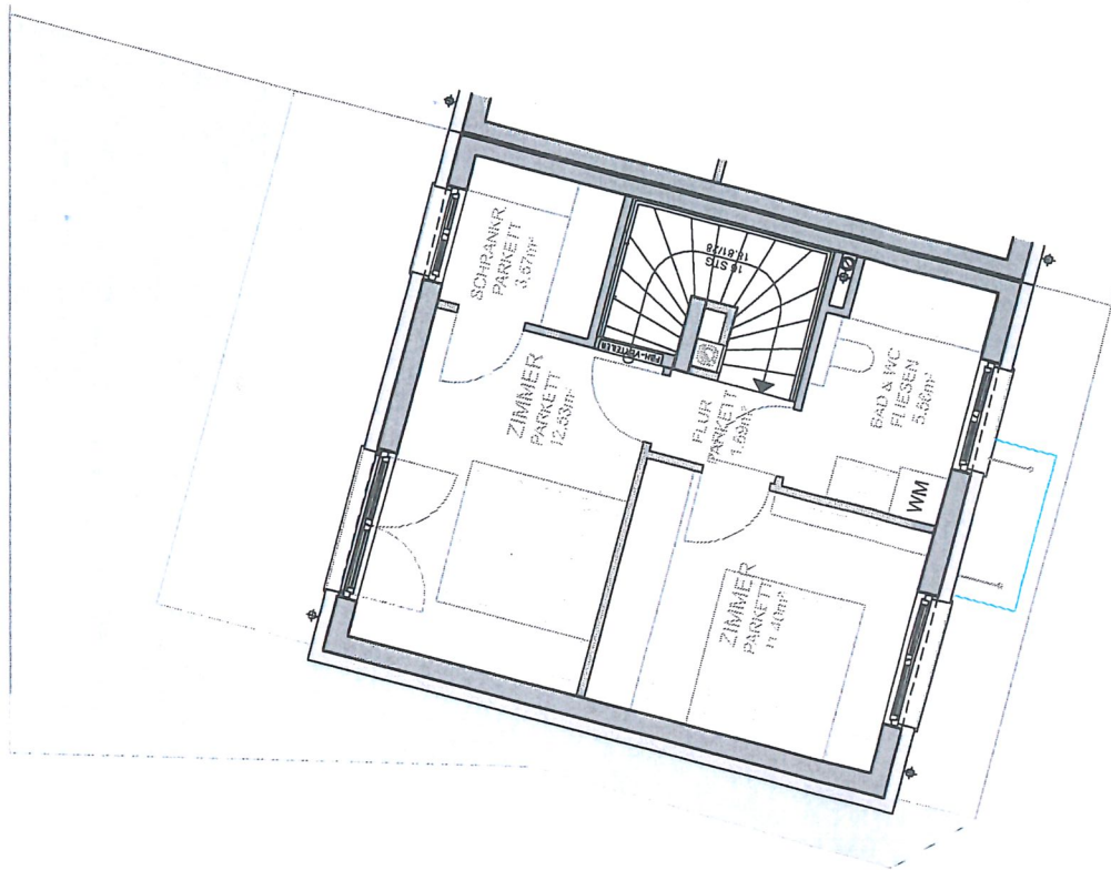
OBERGESCHOSS
