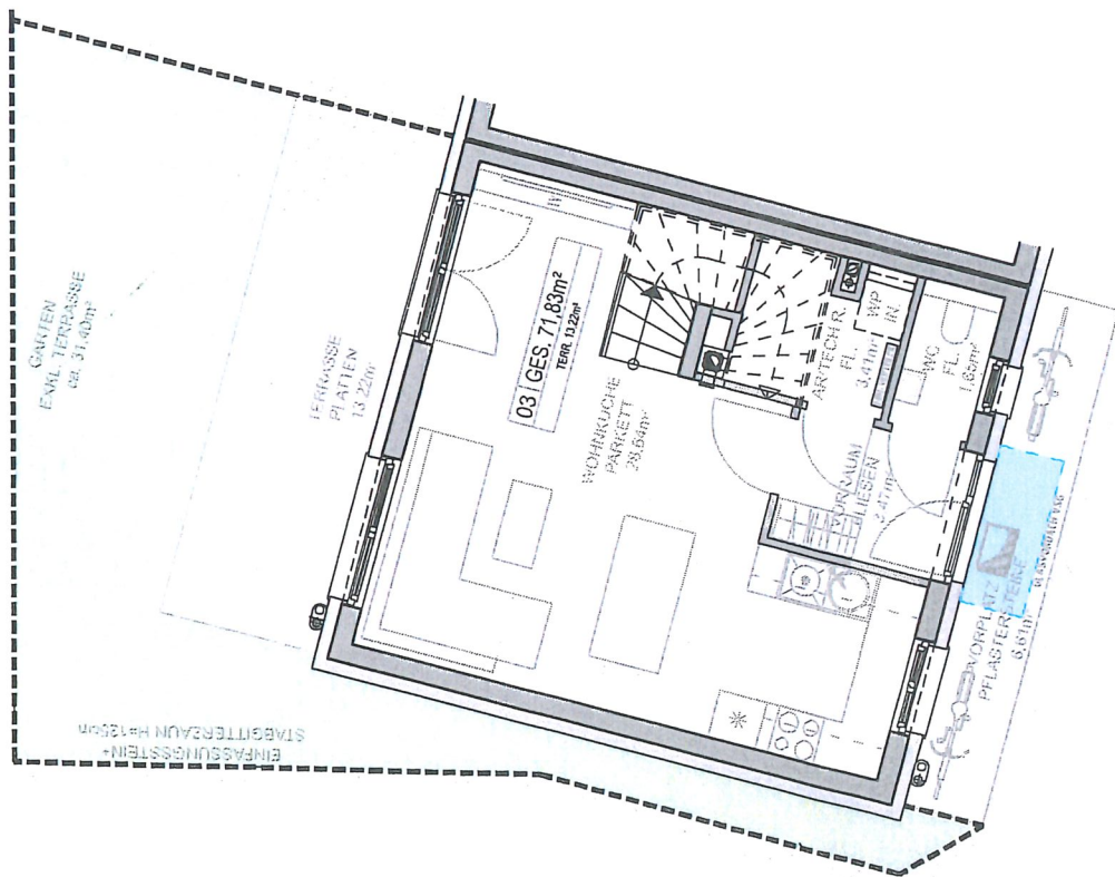
ERDGESCHOSS
