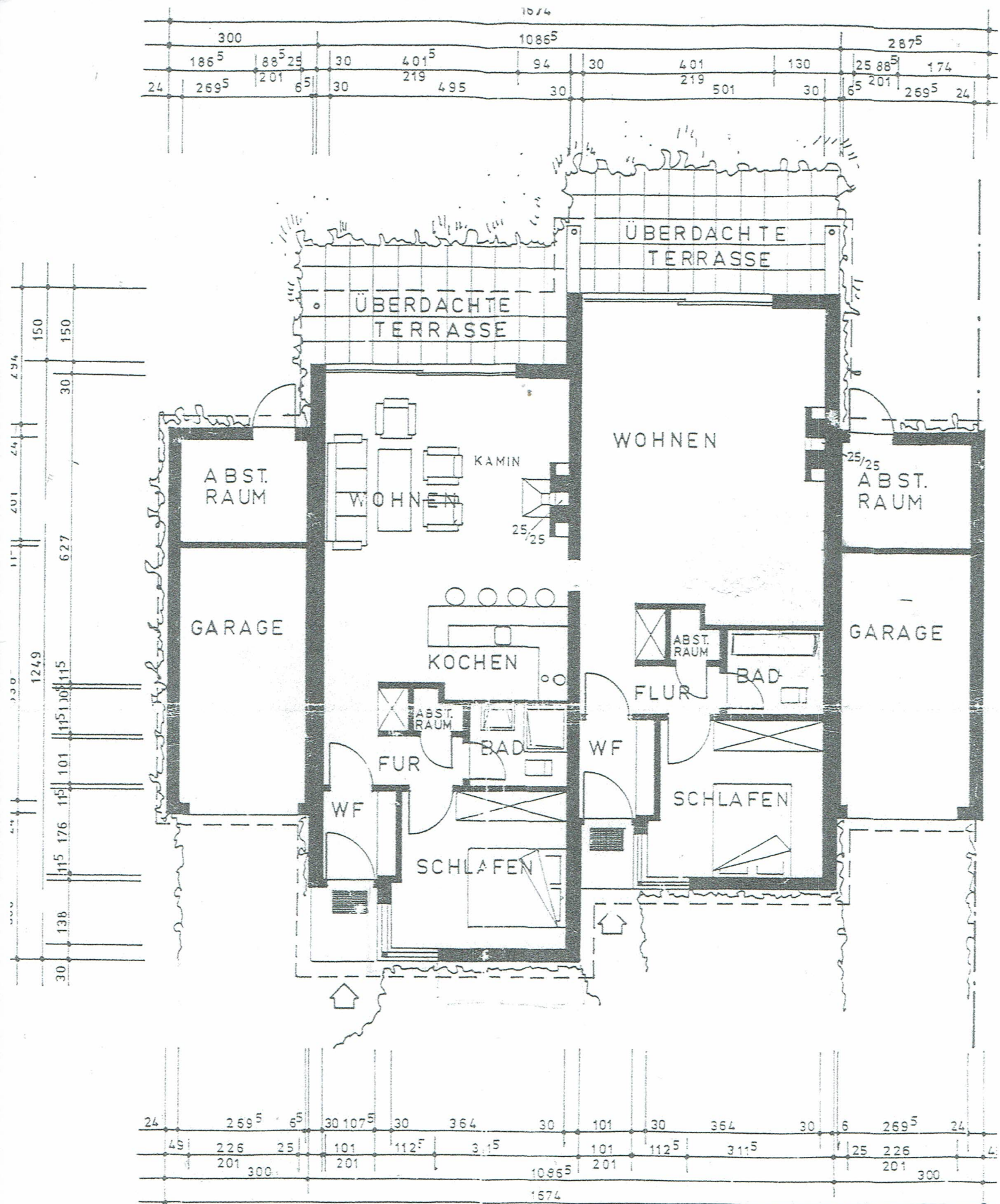
GRUNDRISS M. 1:100
