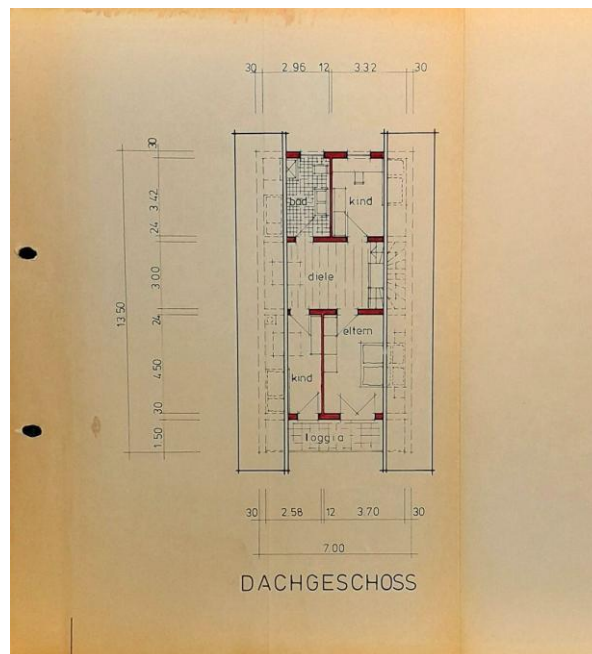
Grundrisse DG
