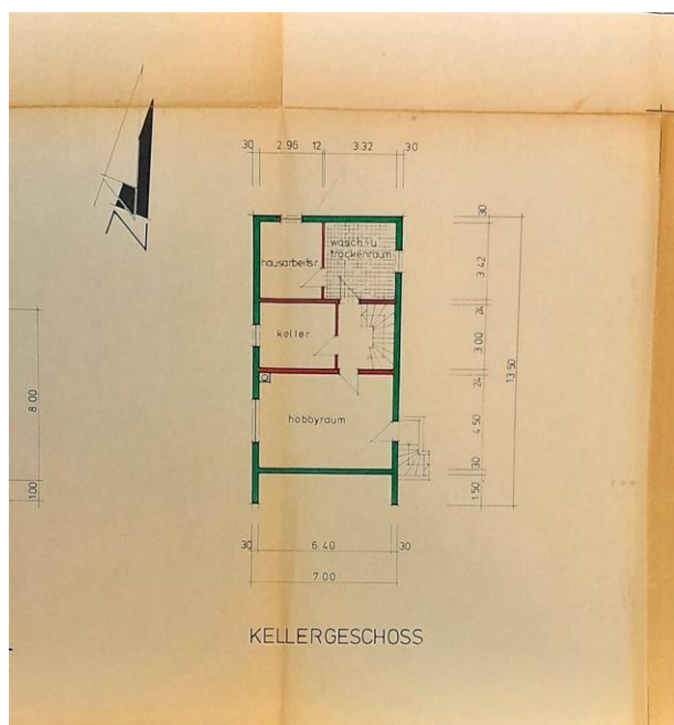
Grundrisse UG
