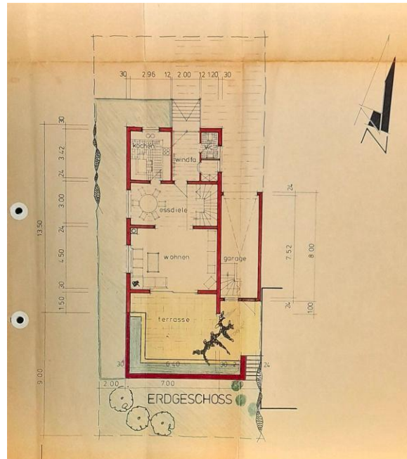
Grundrisse EG
