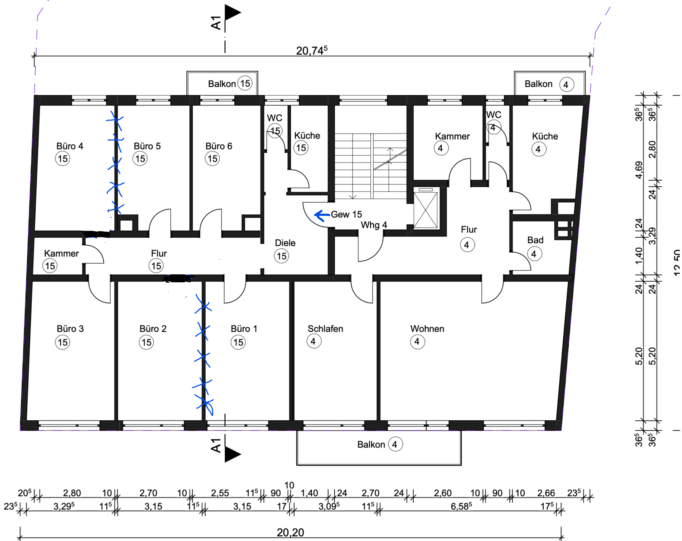
VH 4. OBERGESCHOSS
