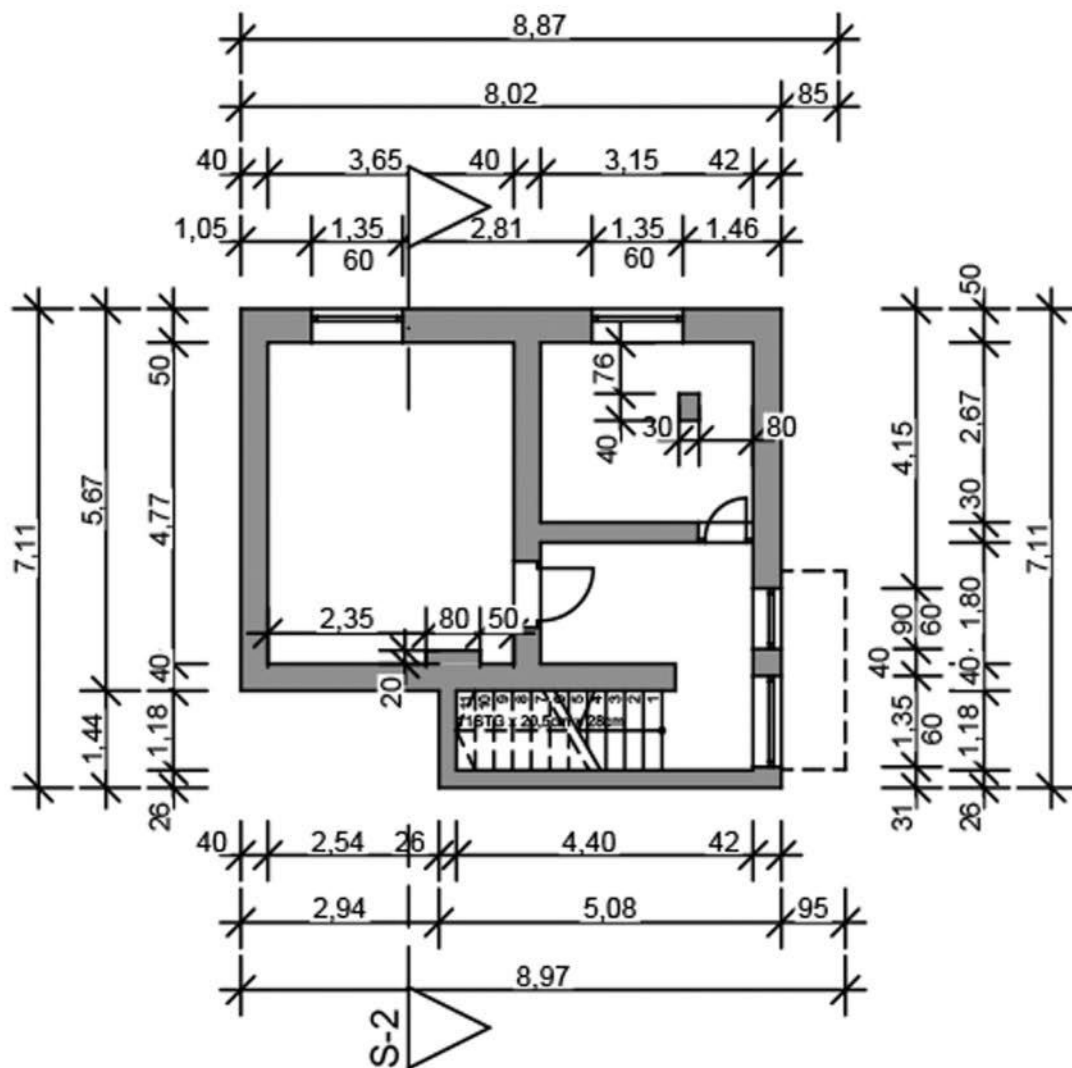
Grundriss Kellergeschoss M 1:200
