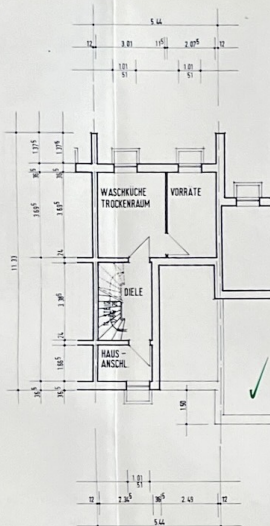
KELLERGESCHOSS
