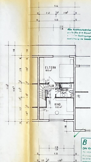
OBERGESCHOSS
