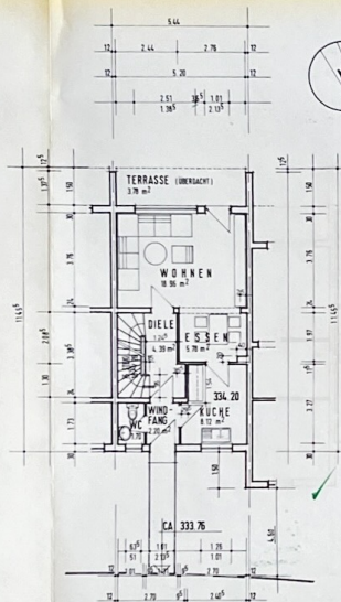
ERDGESCHOSS
