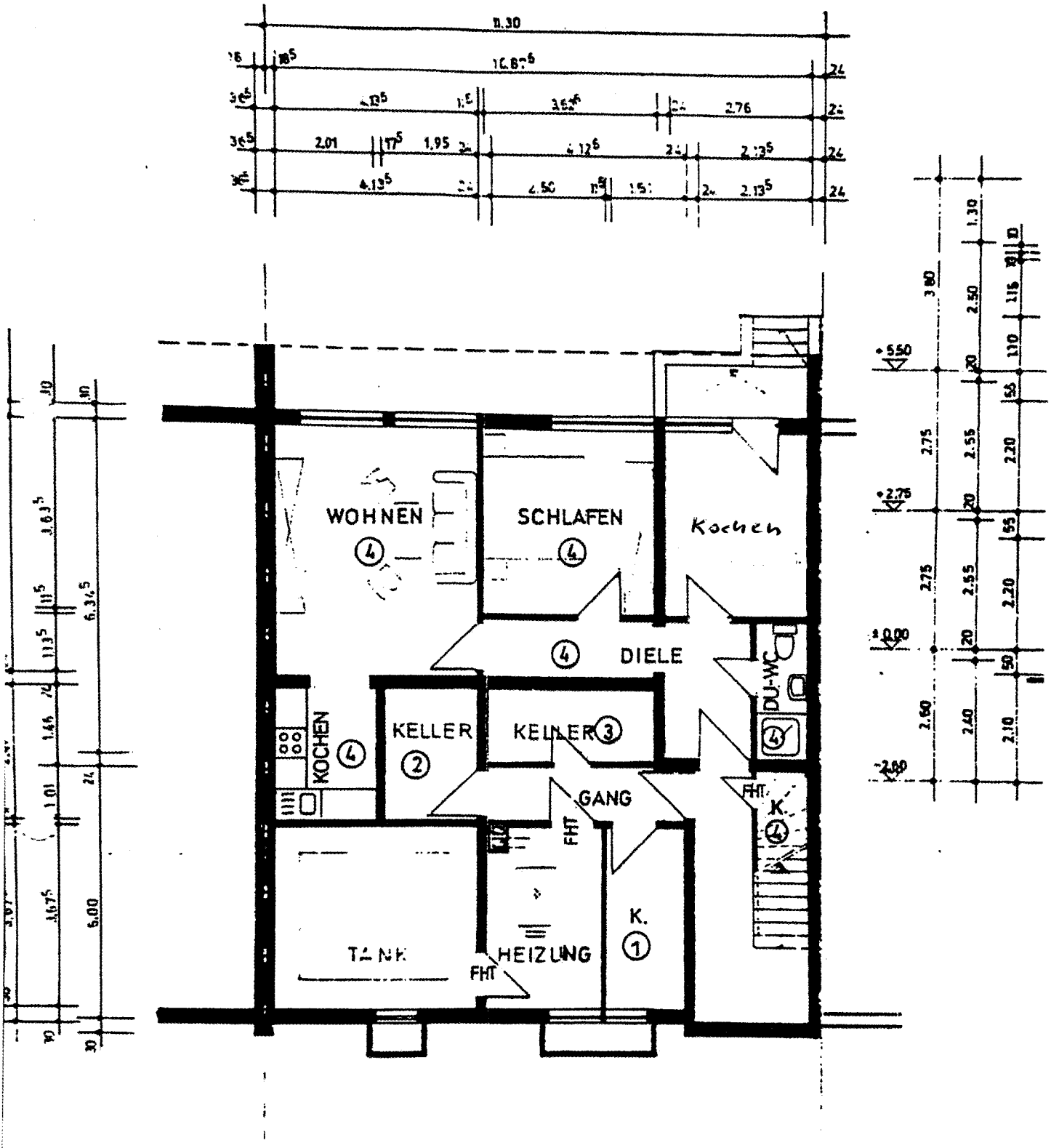
KELLERGESCHOSS
