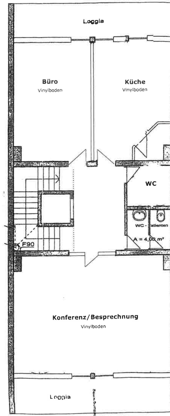
Grundrisszeichnung 3. Obergeschoss (kein Maßstab)
