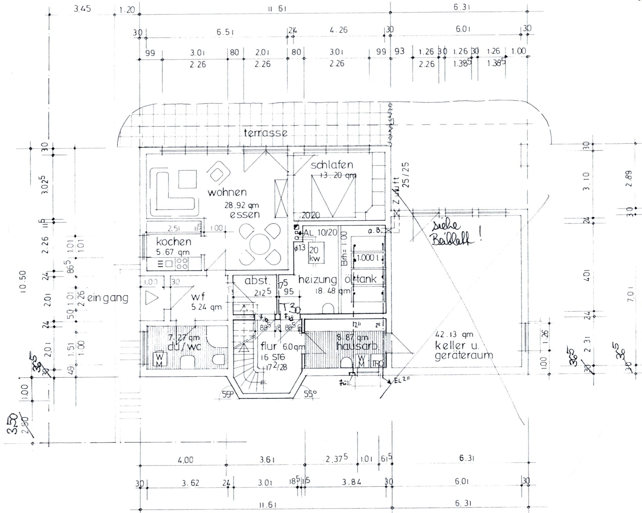
Grundrissplan KG (alt): (nicht maßstabgerecht)
