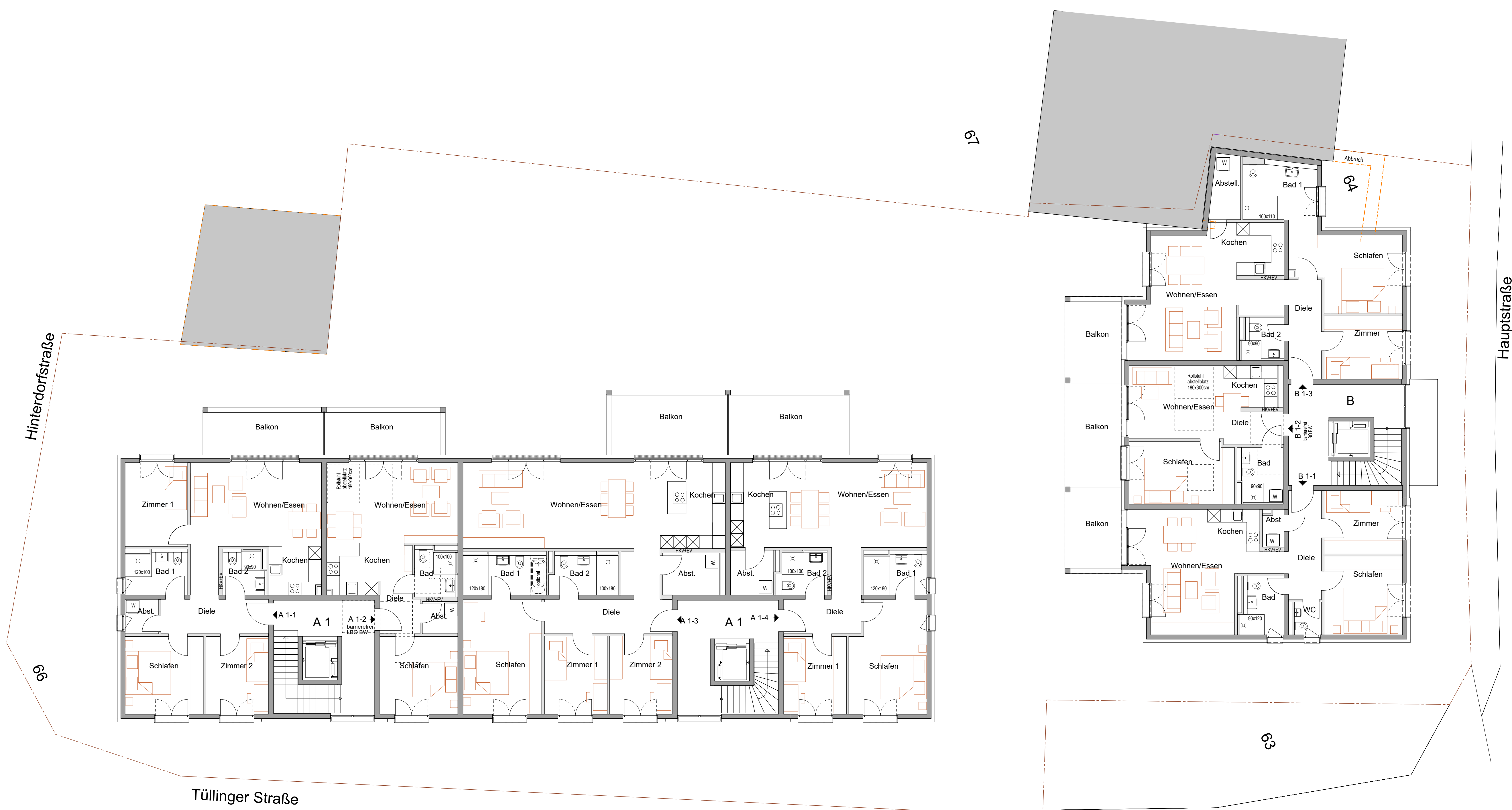
OBERGESCHOSS M. 1:100
