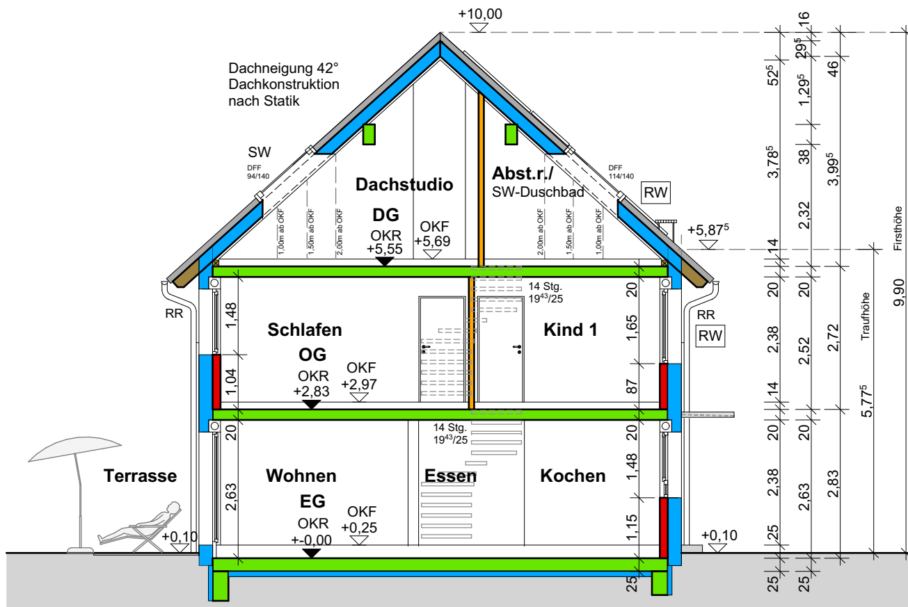
Querschnitt
