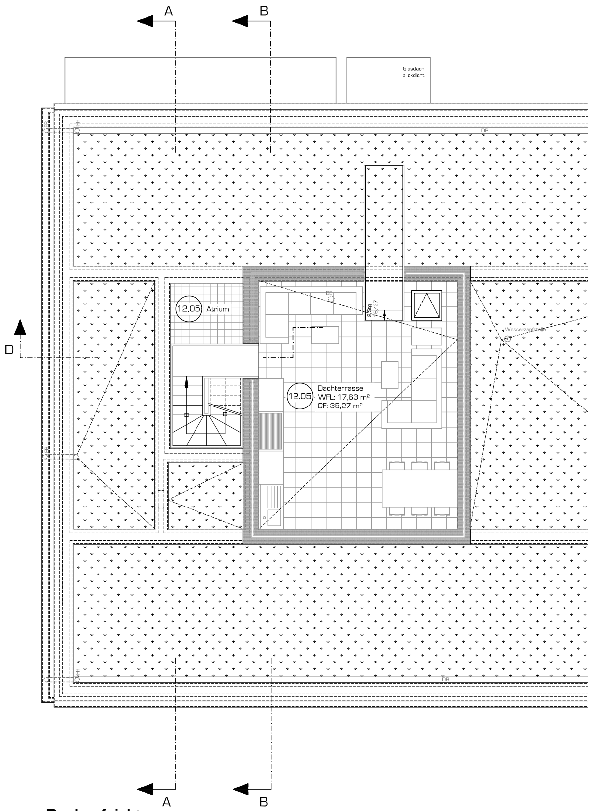
Dachaufsicht
