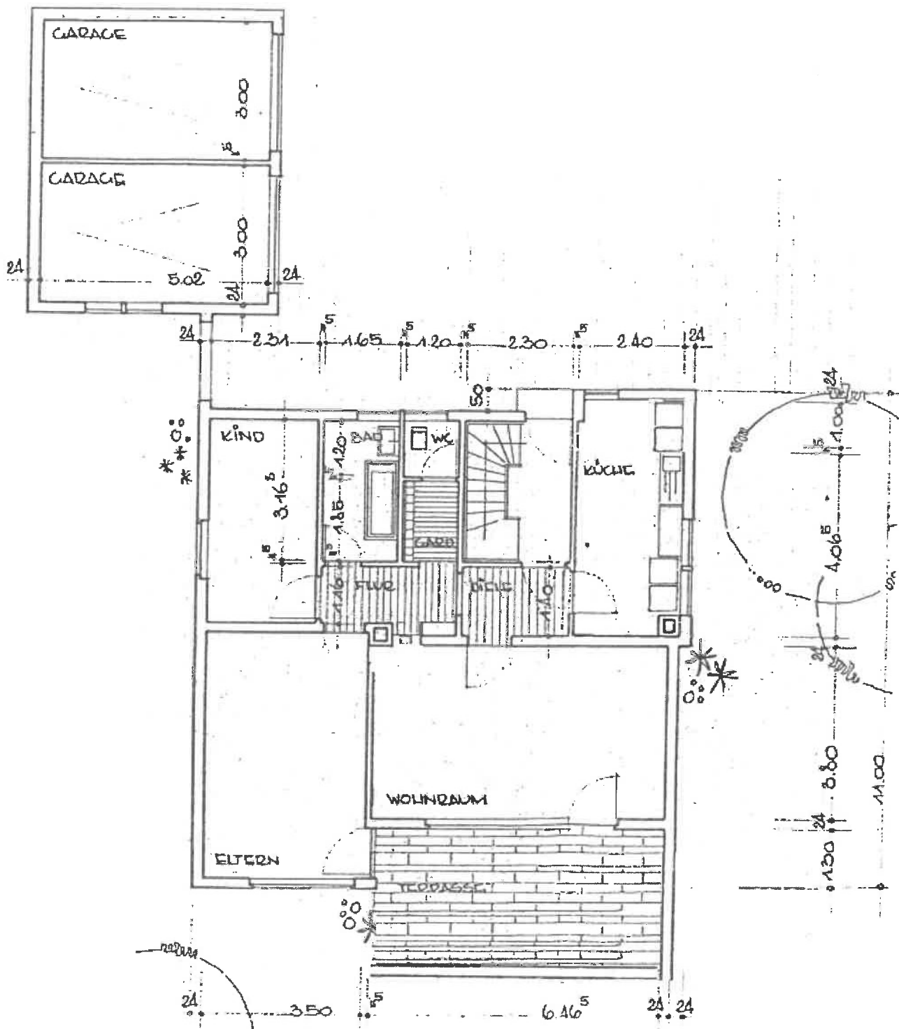
Grundriss Erdgeschoß
