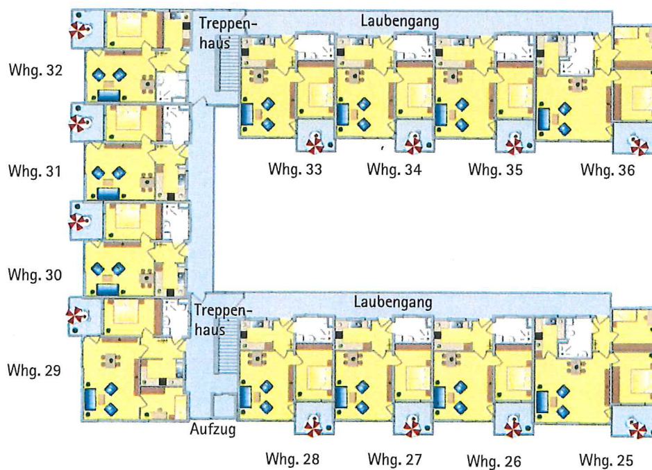
Grundriss 2. Obergeschoss
