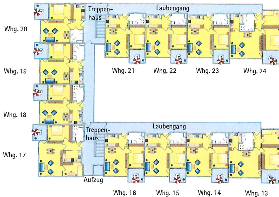
Grundriss 1. Obergeschoss
