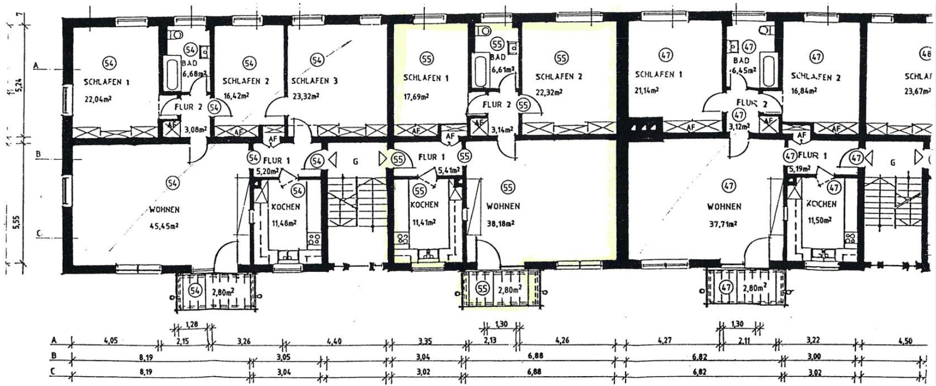
GRUNDRISS 2.OG
