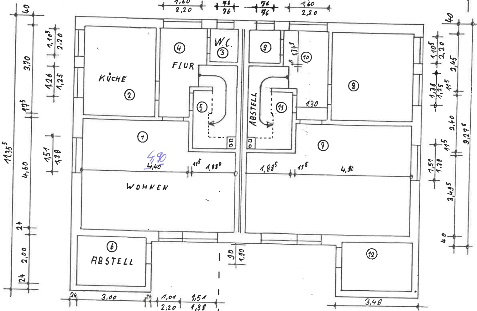
GRUNDRISS
