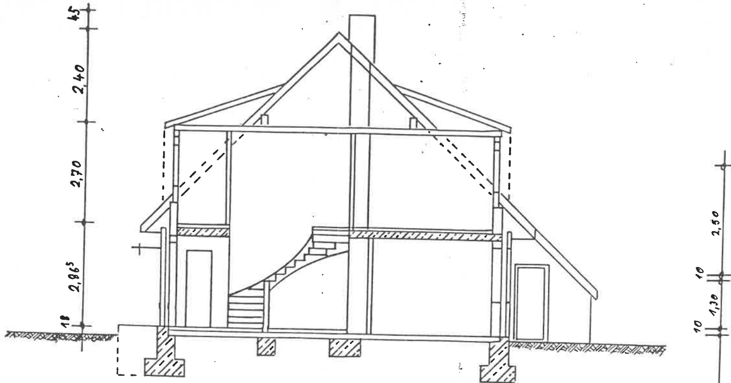
SCHNITT
