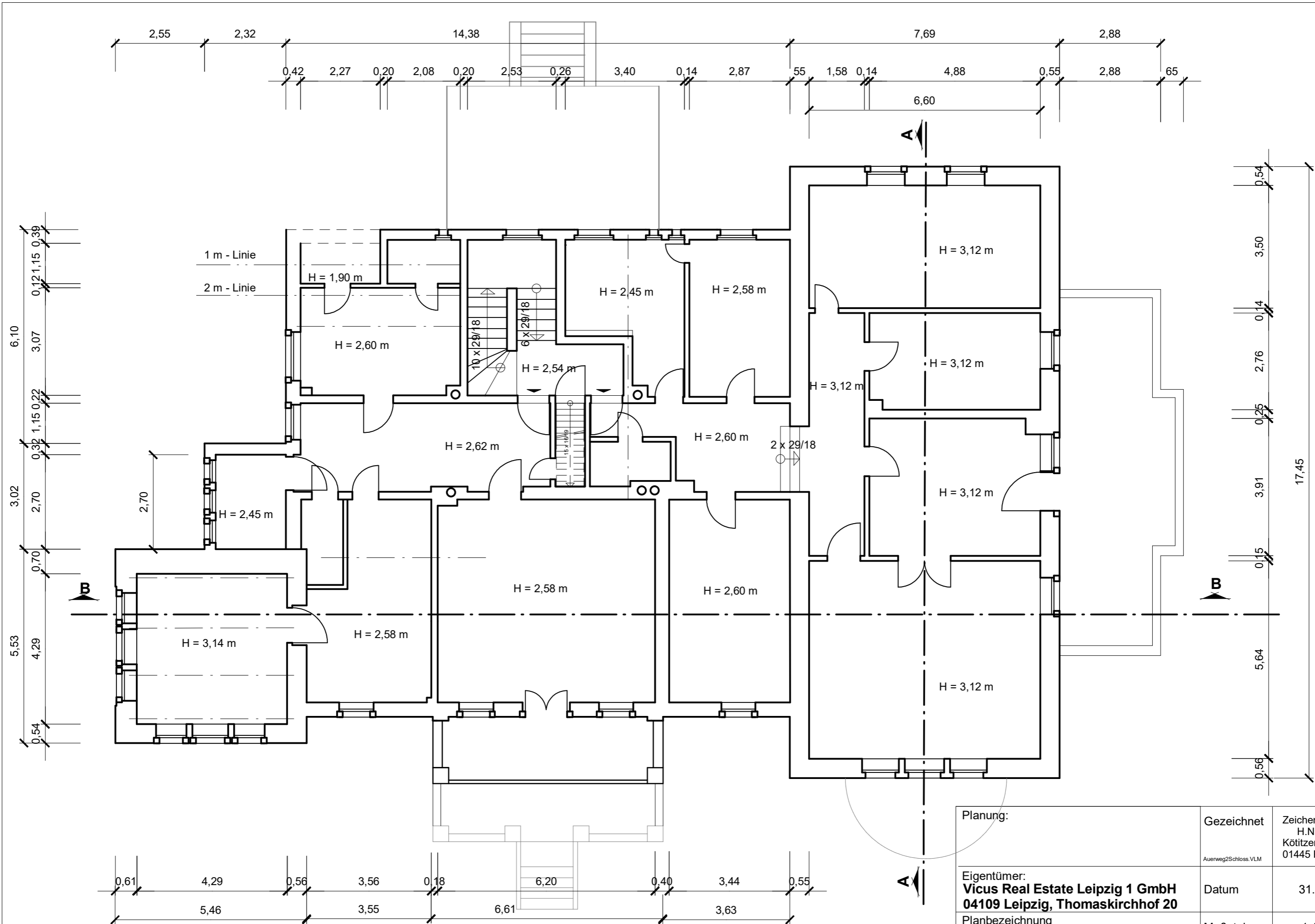
Grundriss OG M 1 : 100
