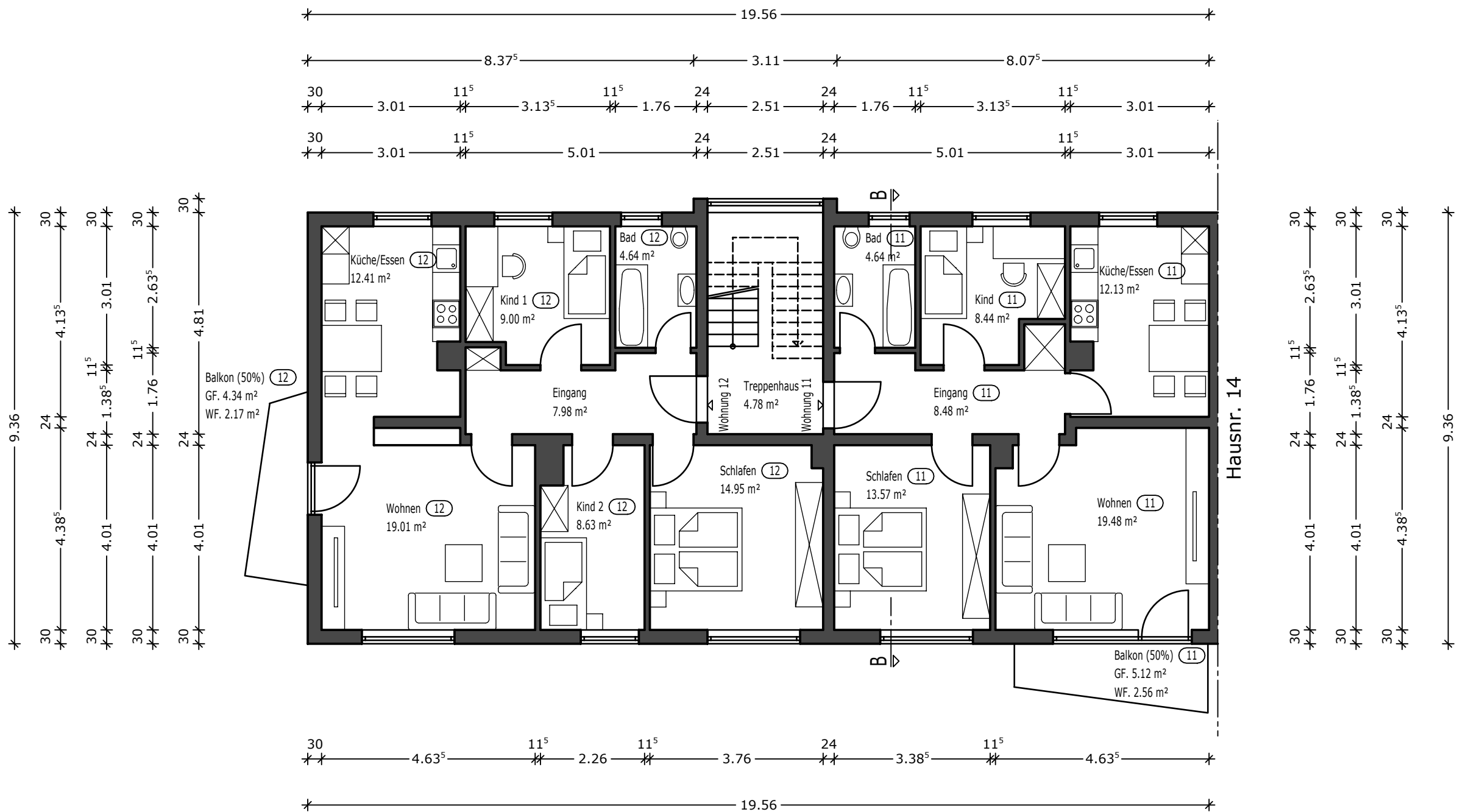
Grundriss 2.Obergeschoss (Hausnummer 16)
