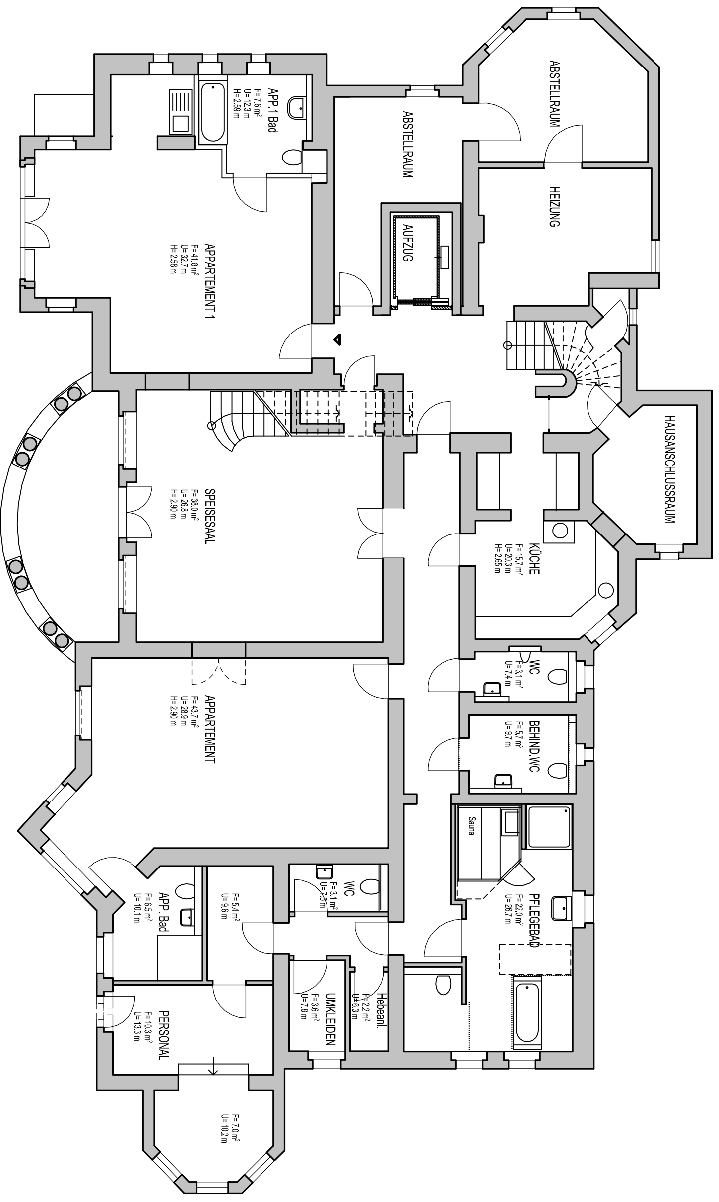
GRUNDRISS SOUTERRAIN M 1: 100 HAUS FELSENECK Fritz - Koch - Str.11, 99817 Eisenach März 2014
