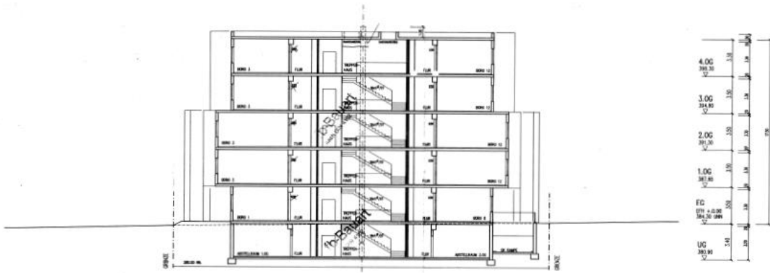
SCHNITT S 1
