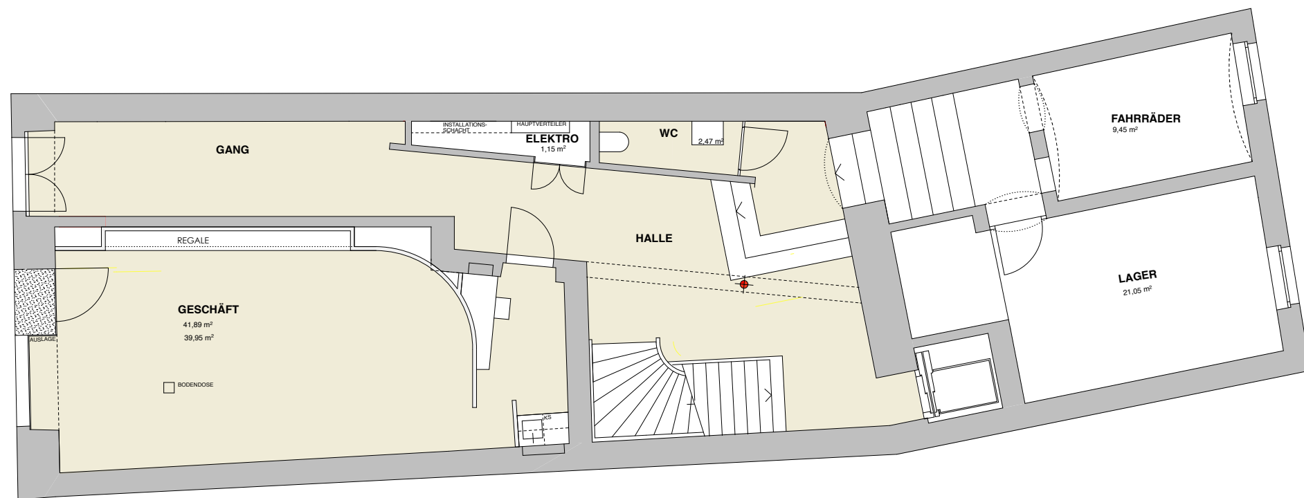
ERDGESCHOSS
