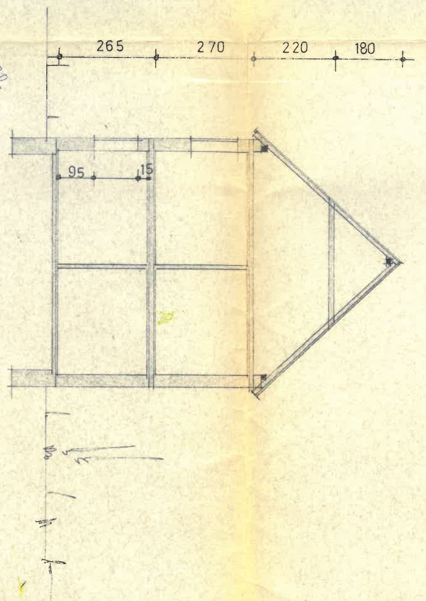
SCHNITT
