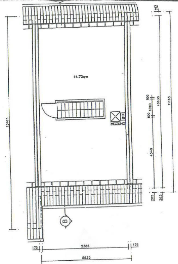
DACHGESCHOSS
