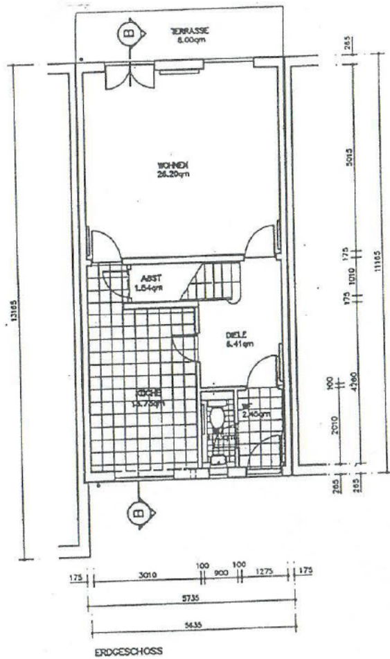
ERDGESCHOSS
