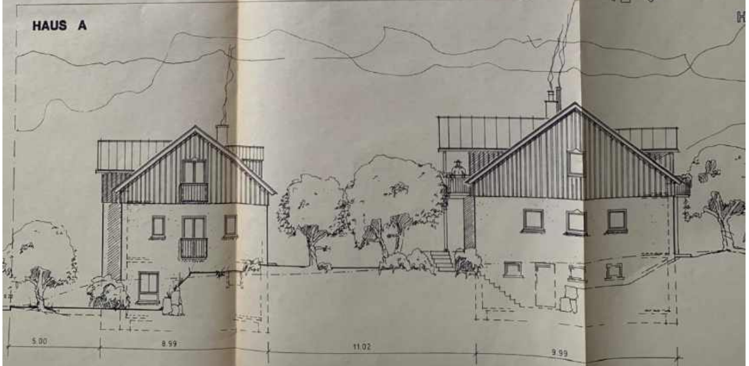
ANSICHT SÜD-OST
