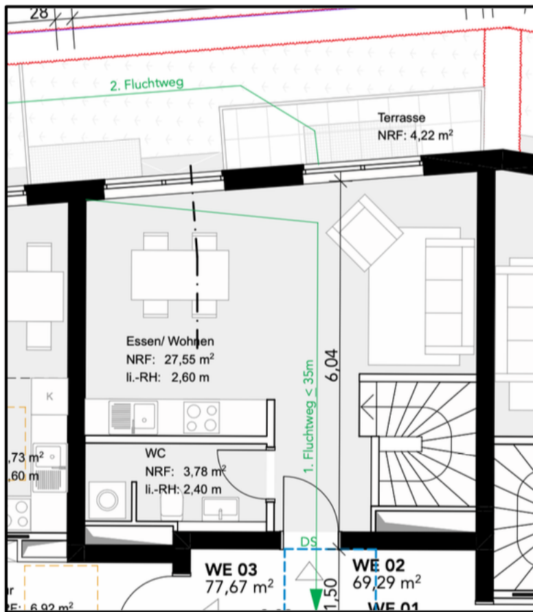
Erdgeschoss
