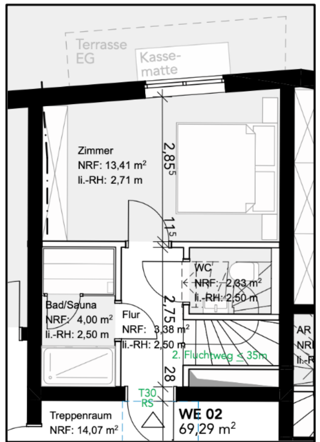
Untergeschoss
