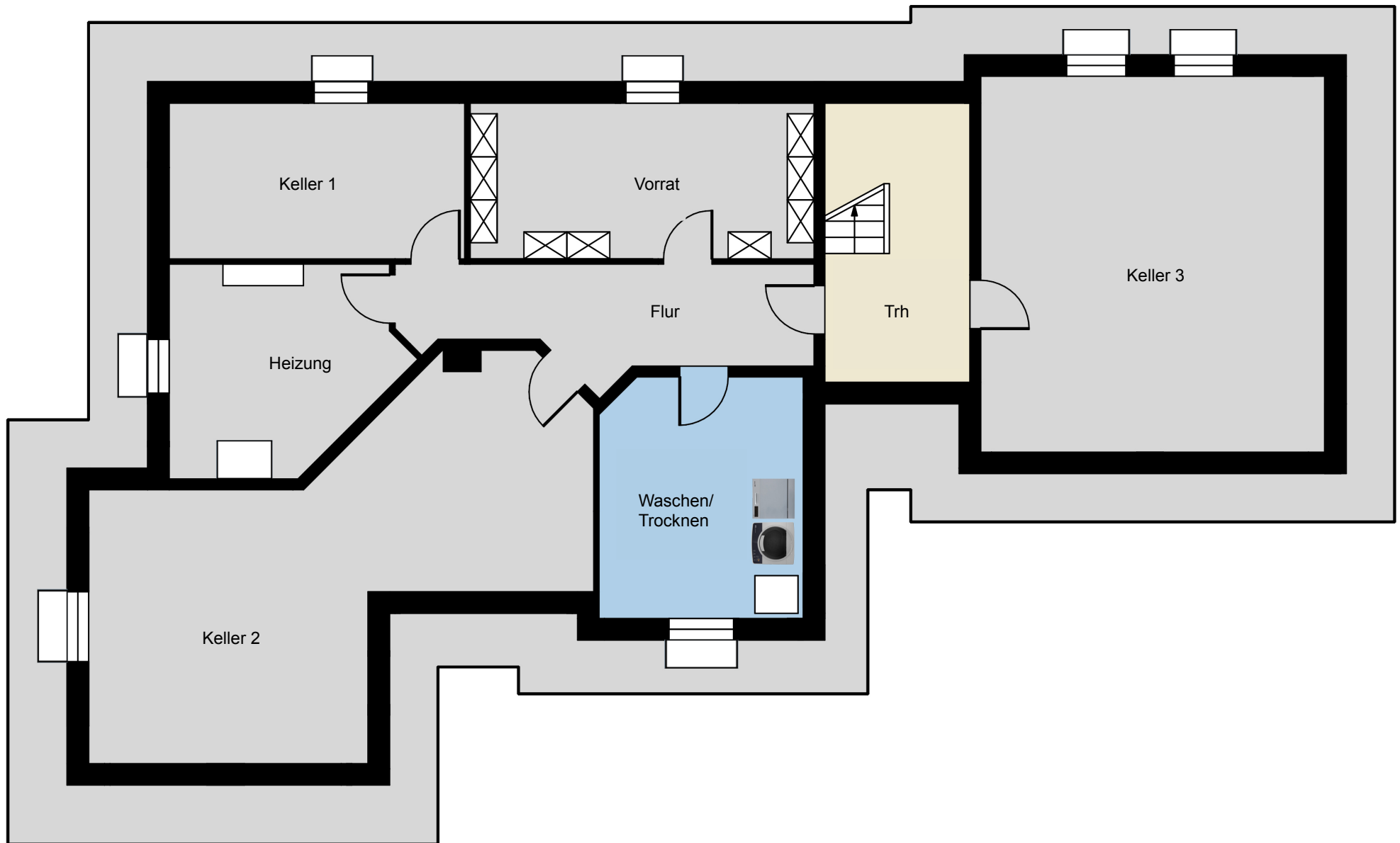
Kellergeschoss
