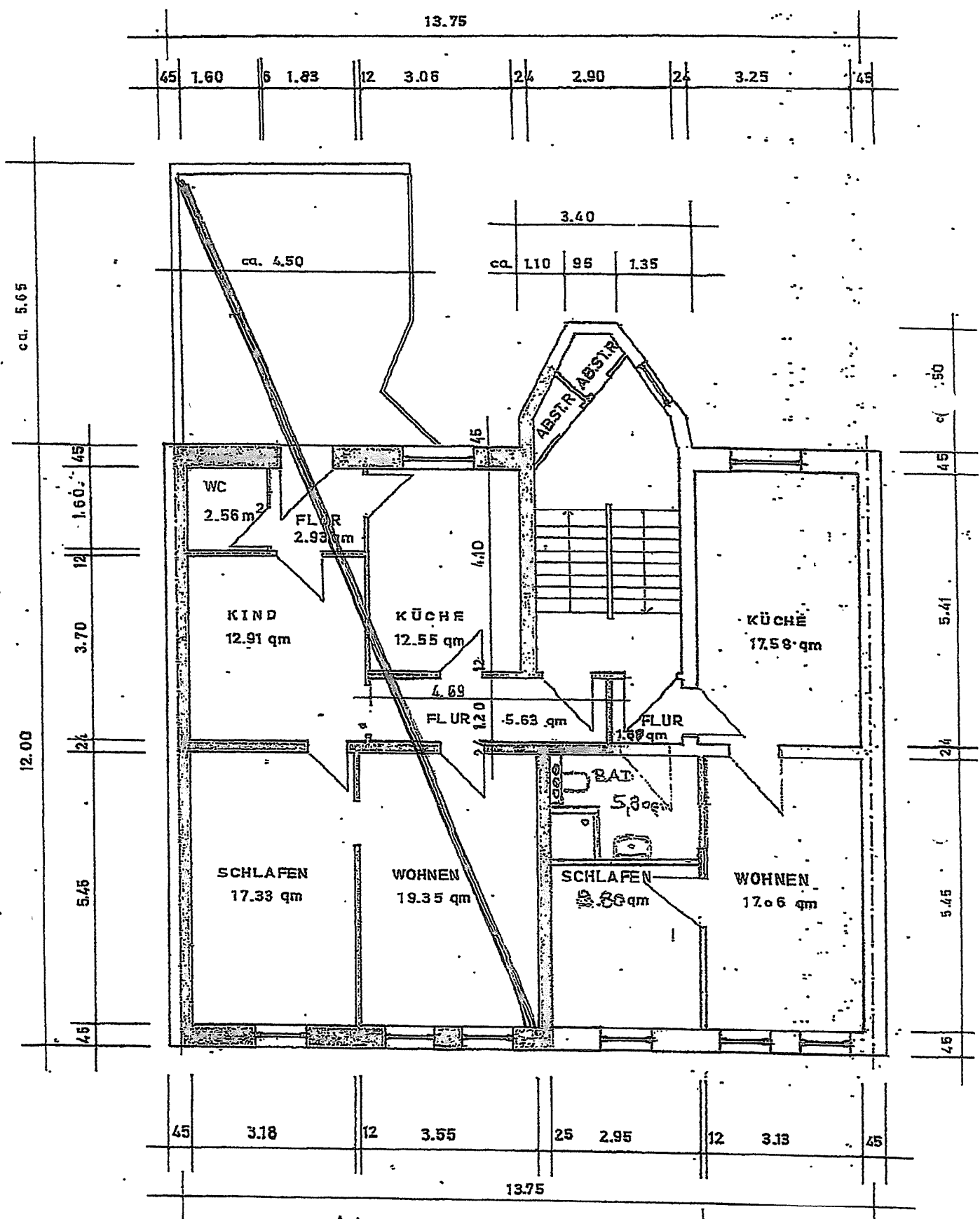
GRUNDRISS 51,00 m 2 BLUMENSTRASSE 3.00 - LINKS
