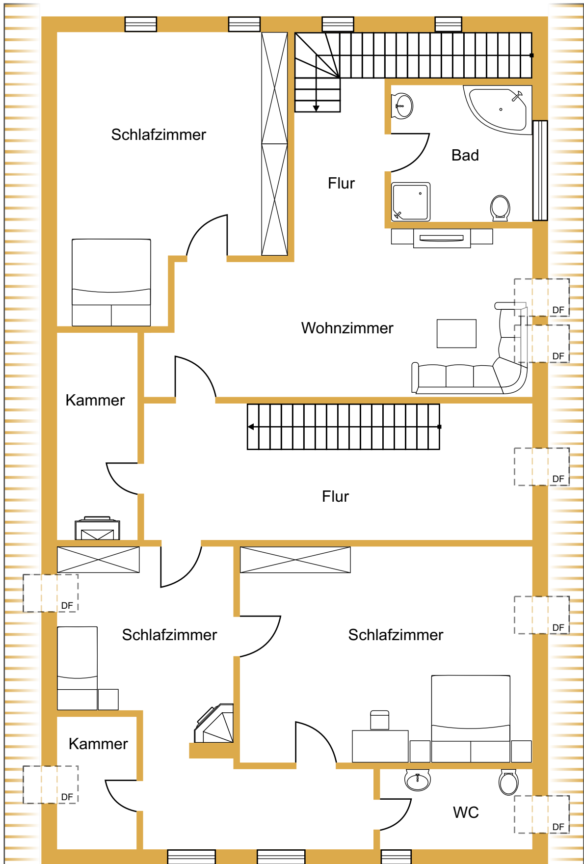
1. Obergeschoss
