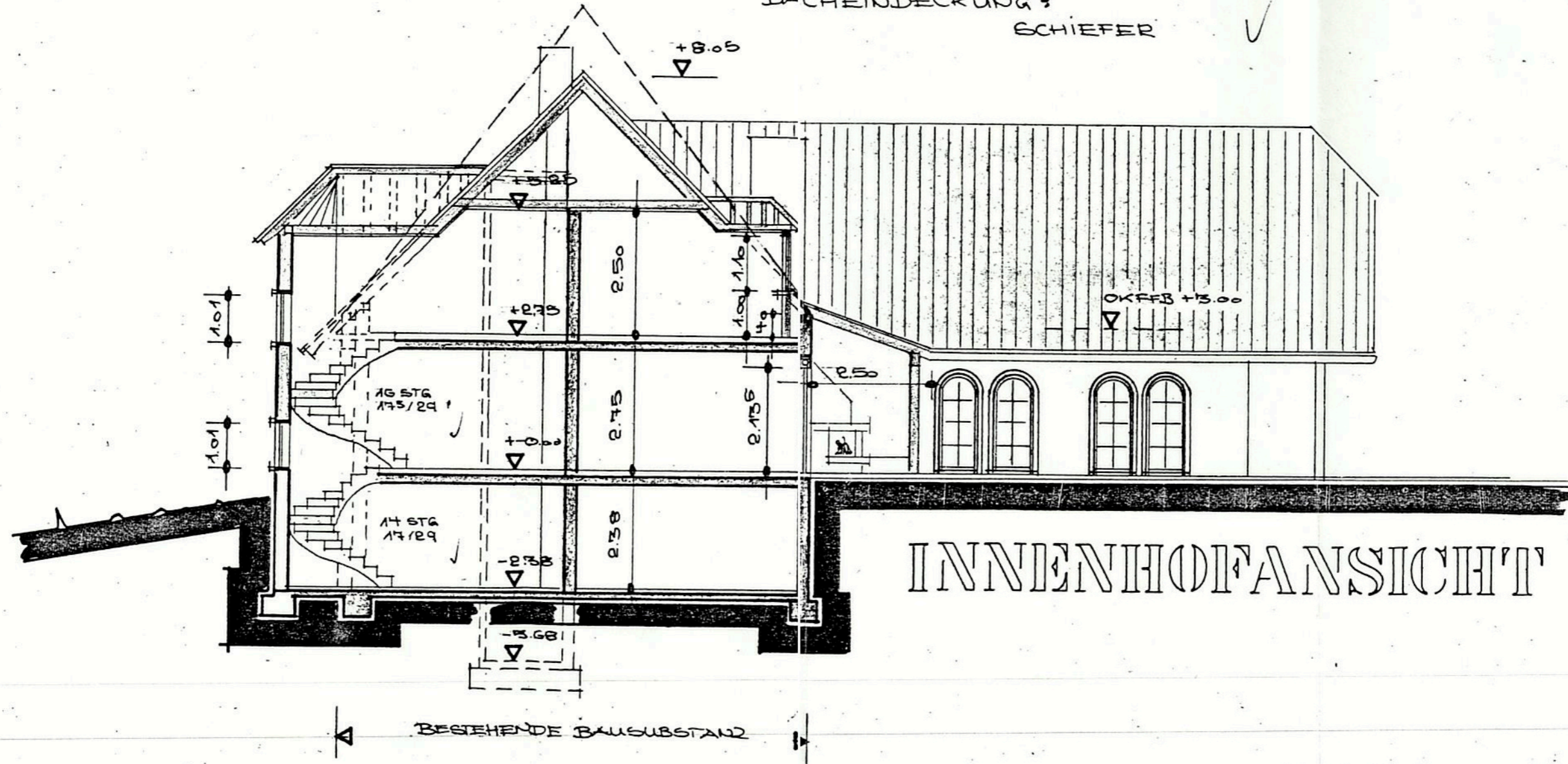
SCHNITT A-A
