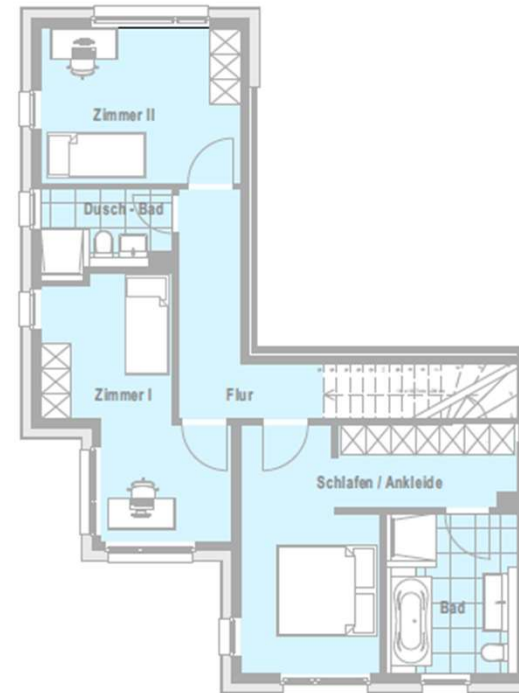
OBERGESCHOSS
