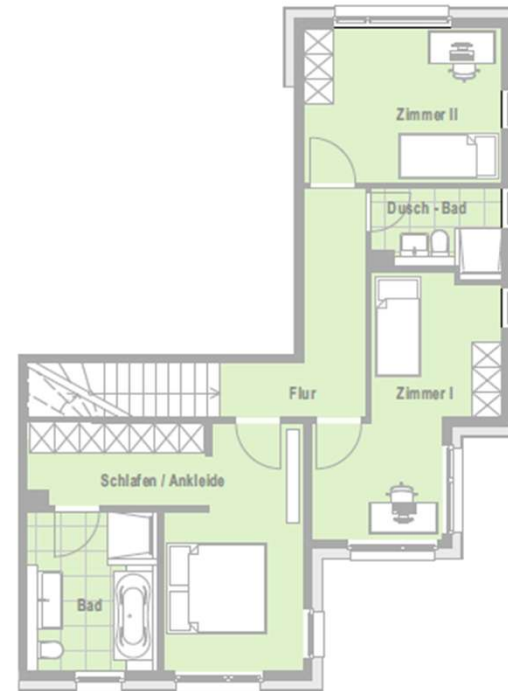
OBERGESCHOSS
