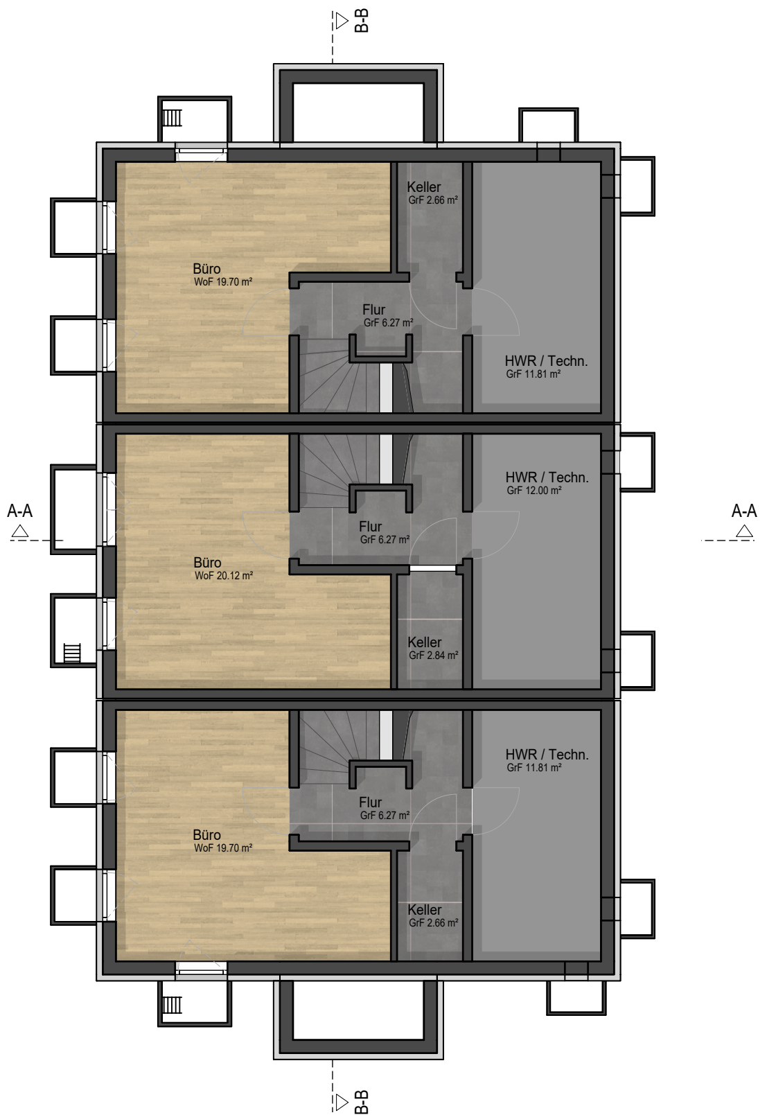
Grundriss KG
